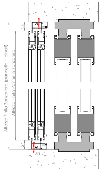
Sezione verticale
