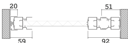
SEZIONE ORIZZONTALE 1 ANTA
