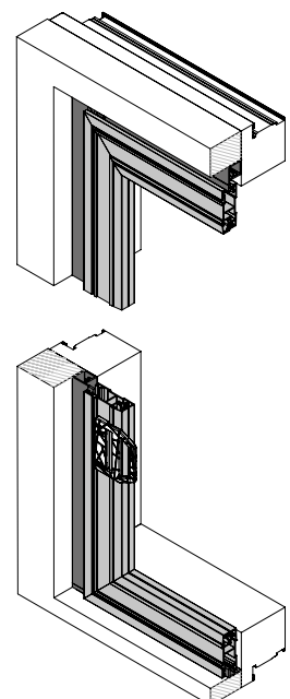
Sezione verticale
