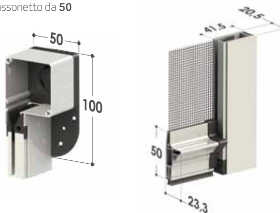
Cassonetto da 50
