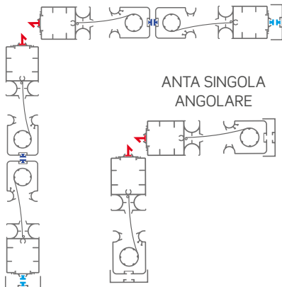
2 ANTE CON APERTURA BILATERALE ANGOLARE
