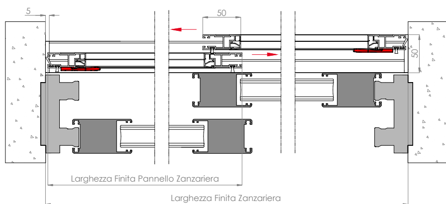
Sezione orizzontale
