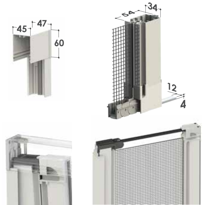
Attacco a baionetta
