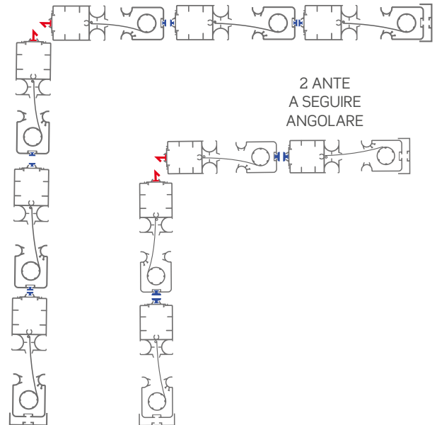
3 ANTE A SEGUIRE ANGOLARE
