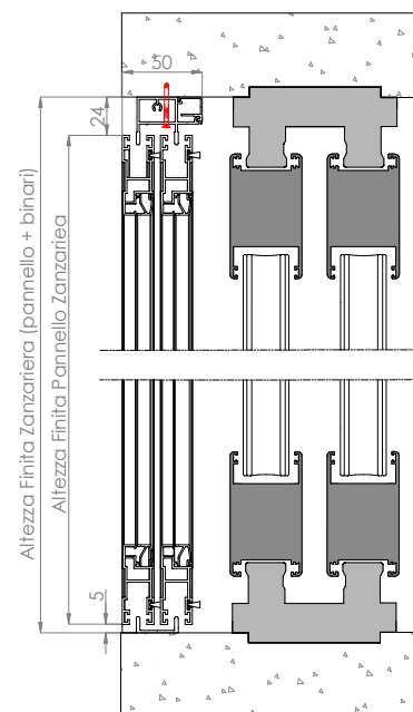
Sezione verticale
