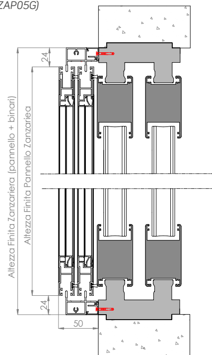
Sezione verticale
