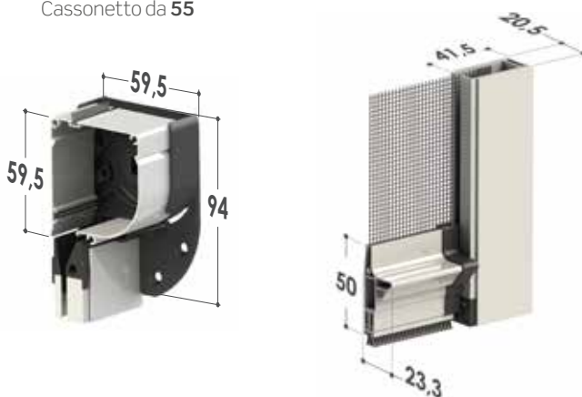
Cassonetto da 55
