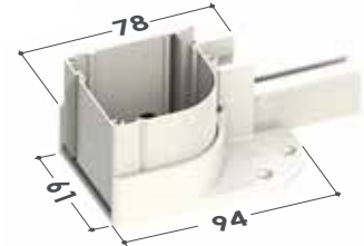
Cassonetto da 55 Testate inferiori
