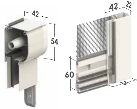
Cassonetto da 42
