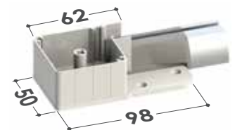
Cassonetto da 50 Testate inferiori
