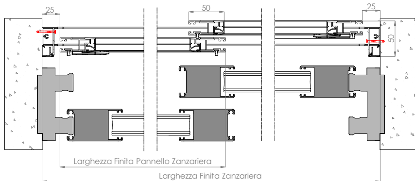
Sezione orizzontale
