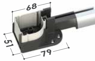
Cassonetto da 45 Testate inferiori
