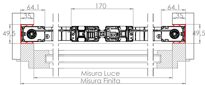
Chiusura centrale
