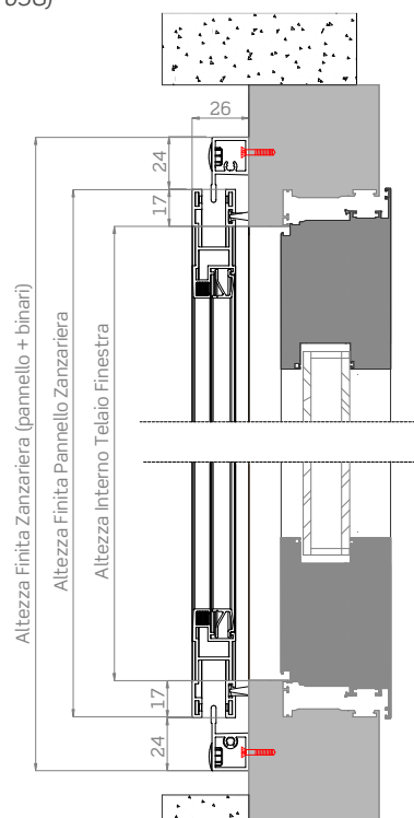
Sezione verticale
