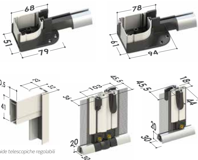
Cassonetto da 45 Testate inferiori
