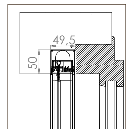
BORA INCAS DOPPIA MIDI 50/50
