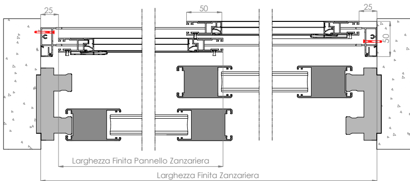
Sezione orizzontale
