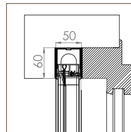
BORA INCAS DOPPIA STANDARD 50/50
