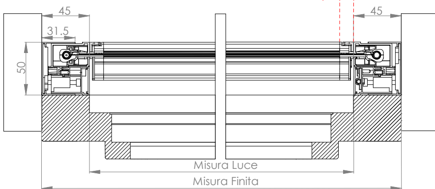
Compensazione fino a 6 mm
