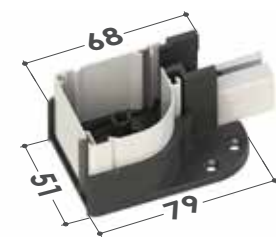
Cassonetto da 45 Testate inferiori
