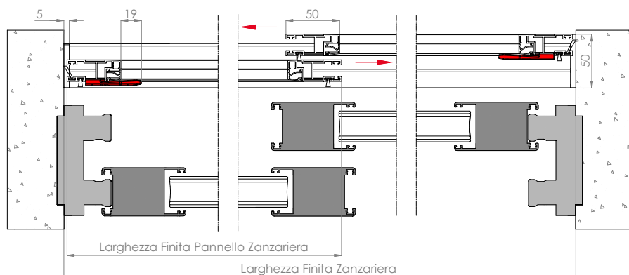
Sezione orizzontale
