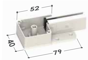
Cassonetto da 40 Testate inferiori
