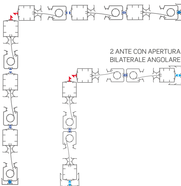
3 ANTE A SEGUIRE ANGOLARE
