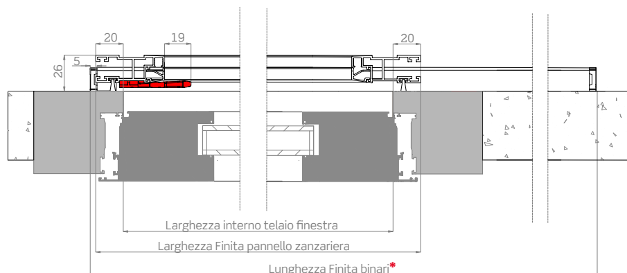
Sezione orizzontale
