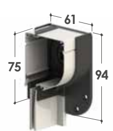
Cassonetto da 55
