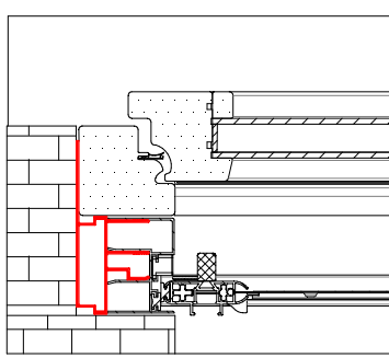
SEZIONE ORIZZONTALE
