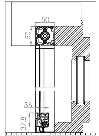
IRINA INSTALLAZIONE A INCASSO
