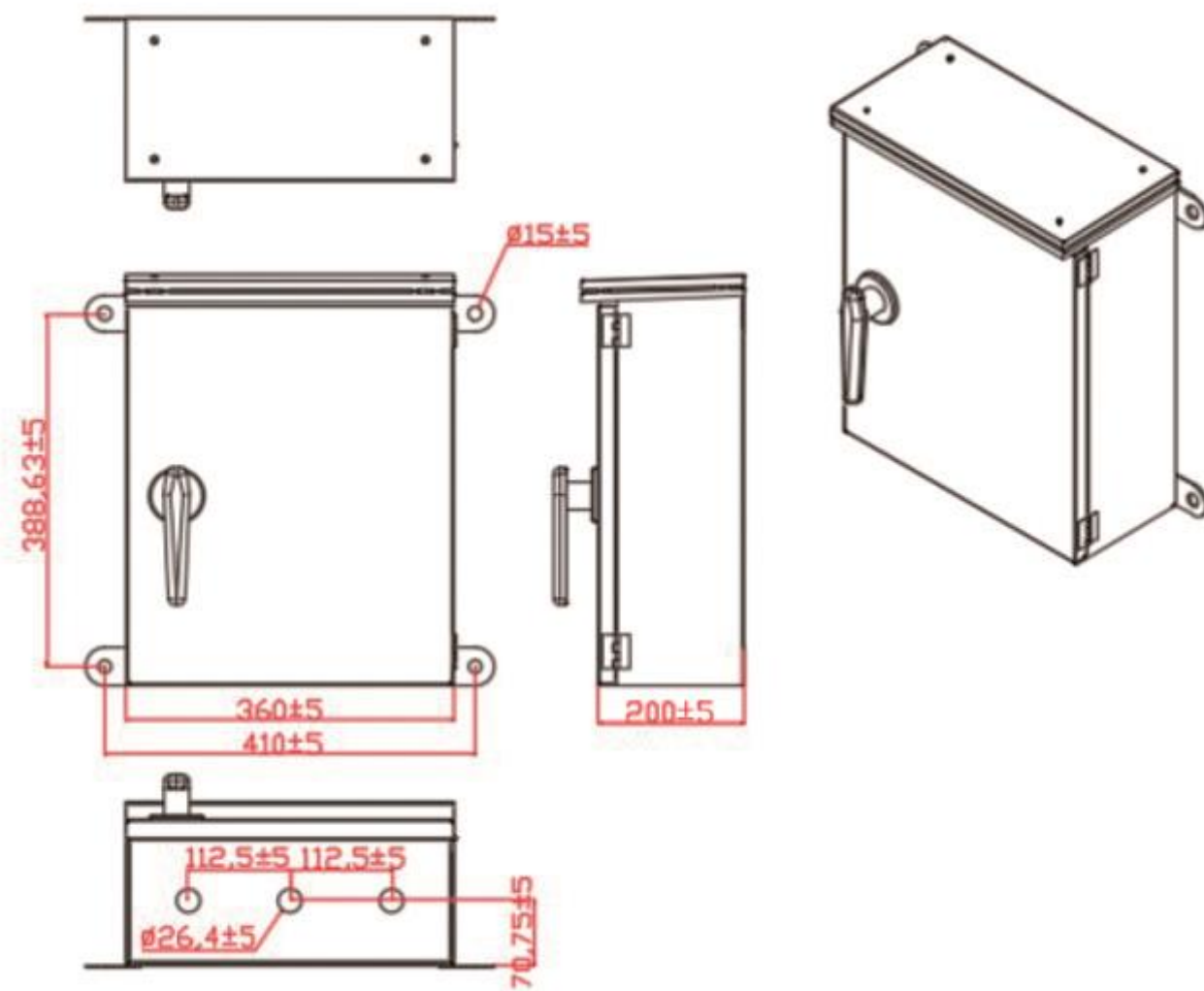
監控箱尺寸 (單位=mm)
