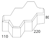
Esse 80 220x110x80mm
