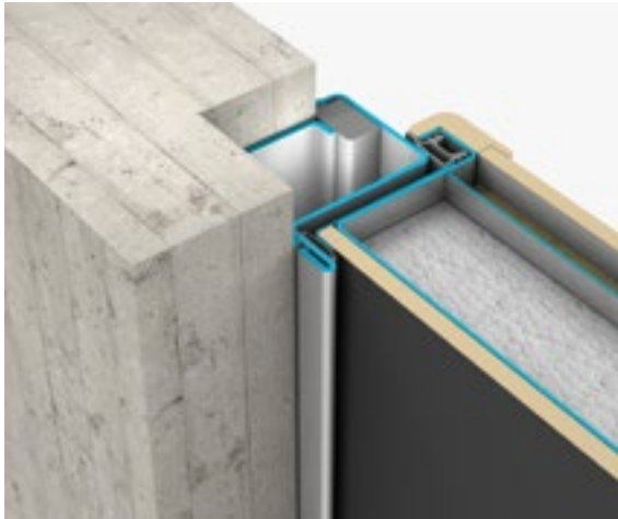
3 Soluzione telaio G standard senza profili di copertura telaio
