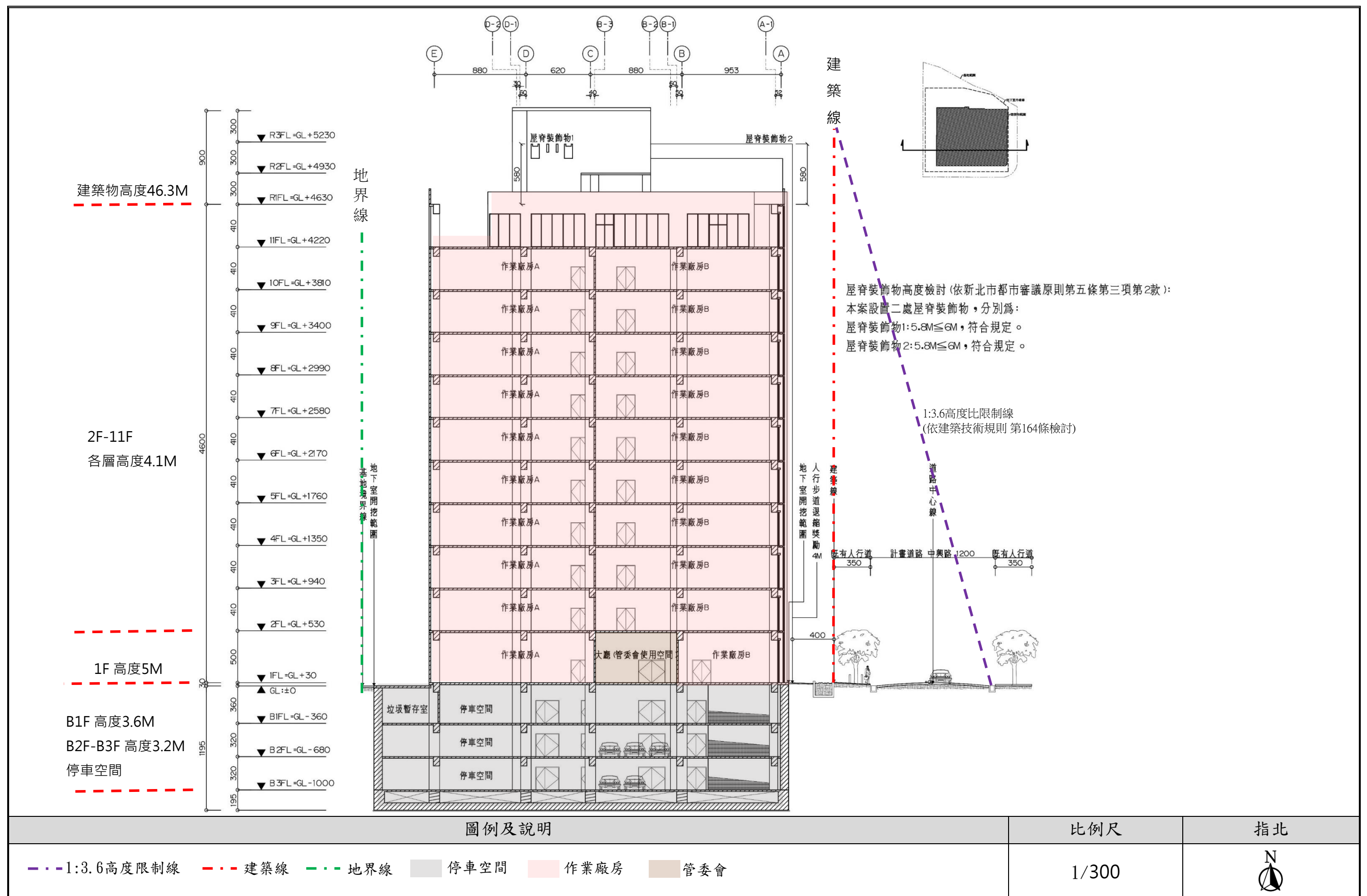
圖11-28 縱向剖面圖
