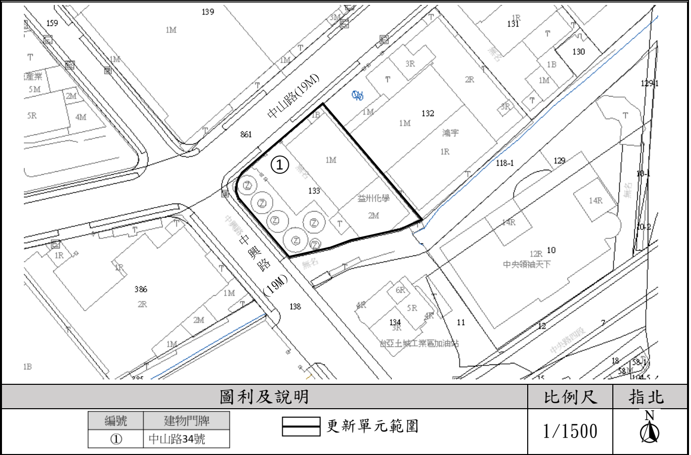
圖5-2 合法建築物門牌座落位置示意圖
