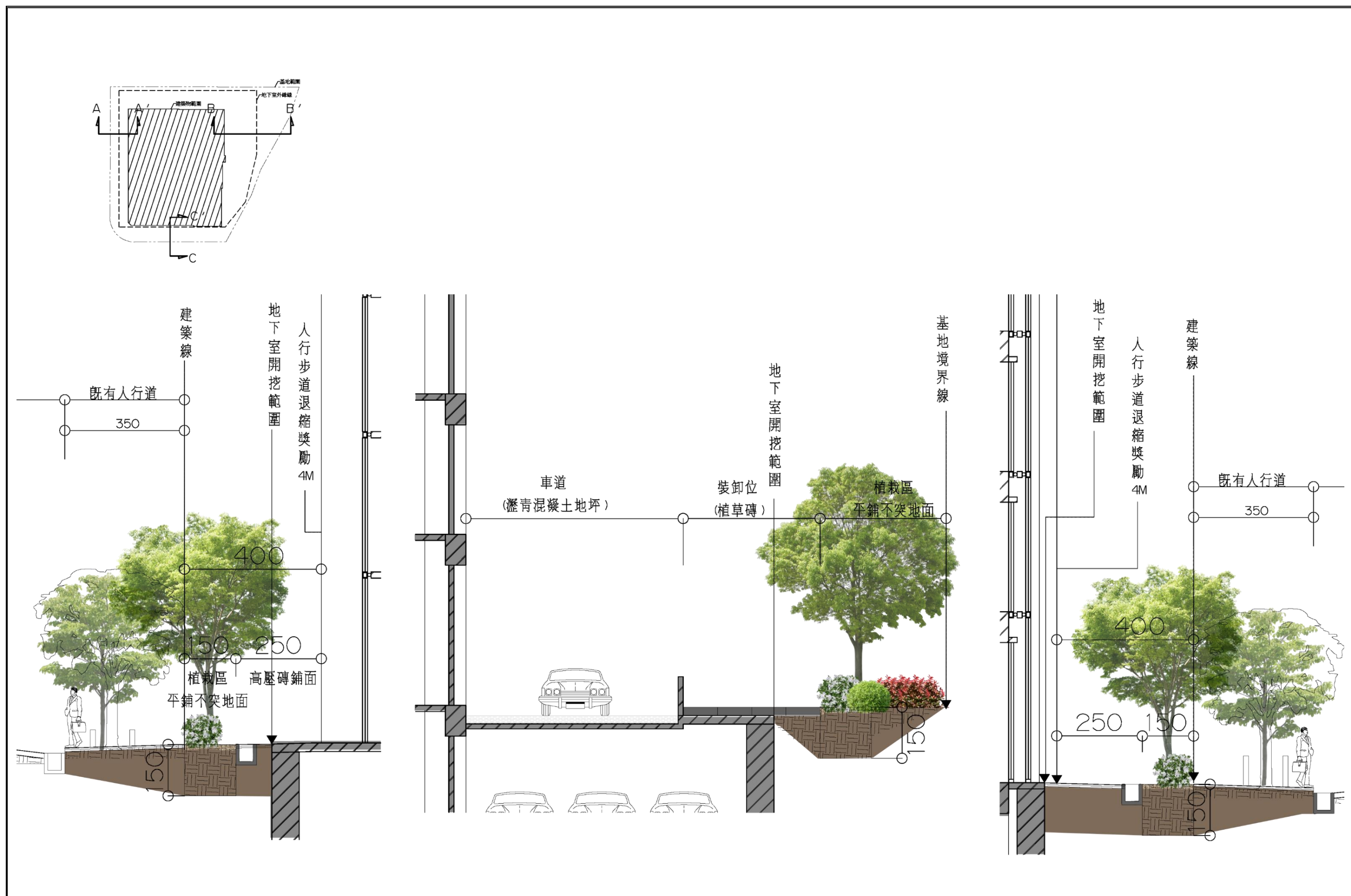
圖12-28 景觀剖面圖
