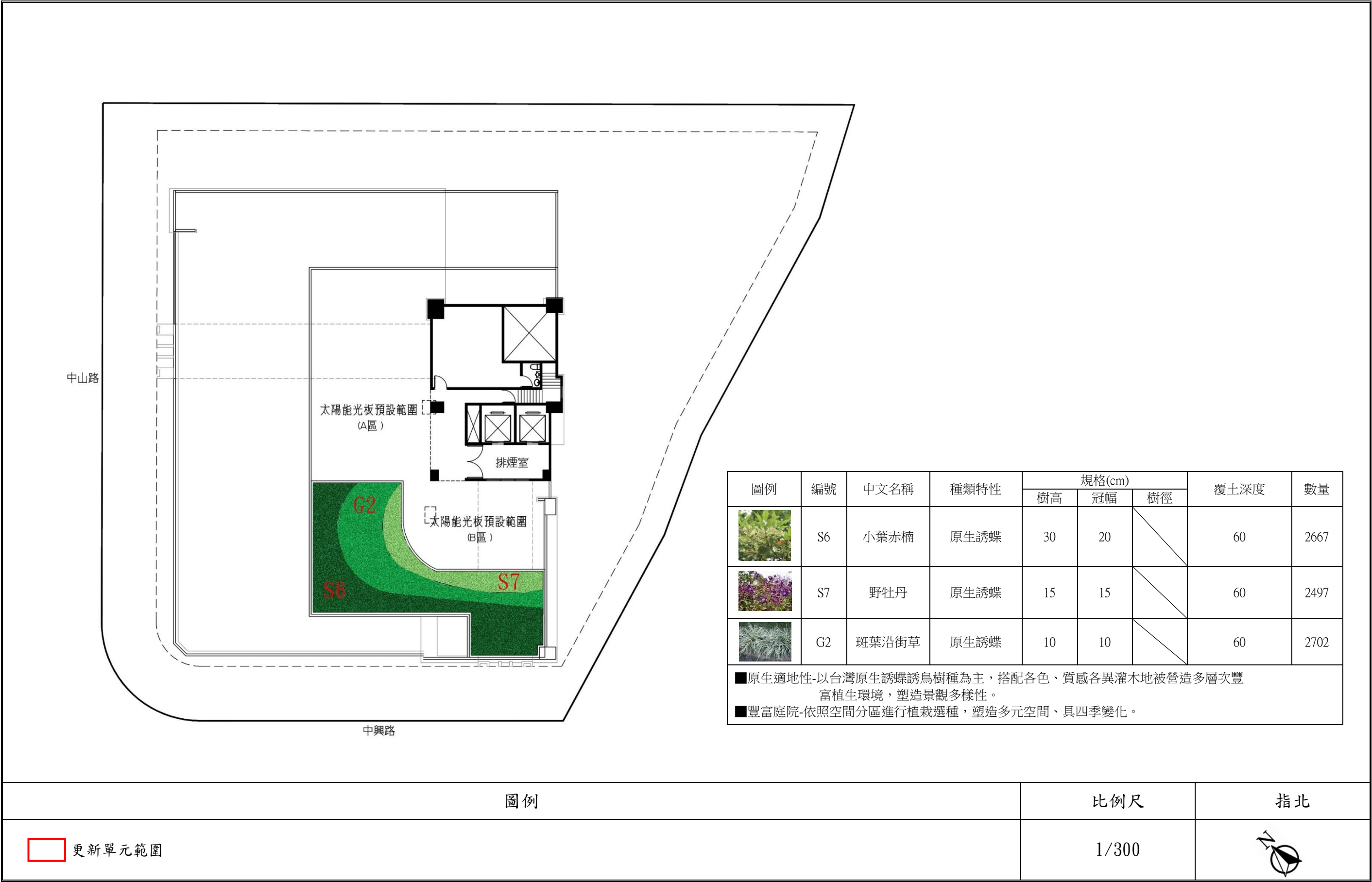
圖12-24 屋頂層景觀灌木植栽配置圖
