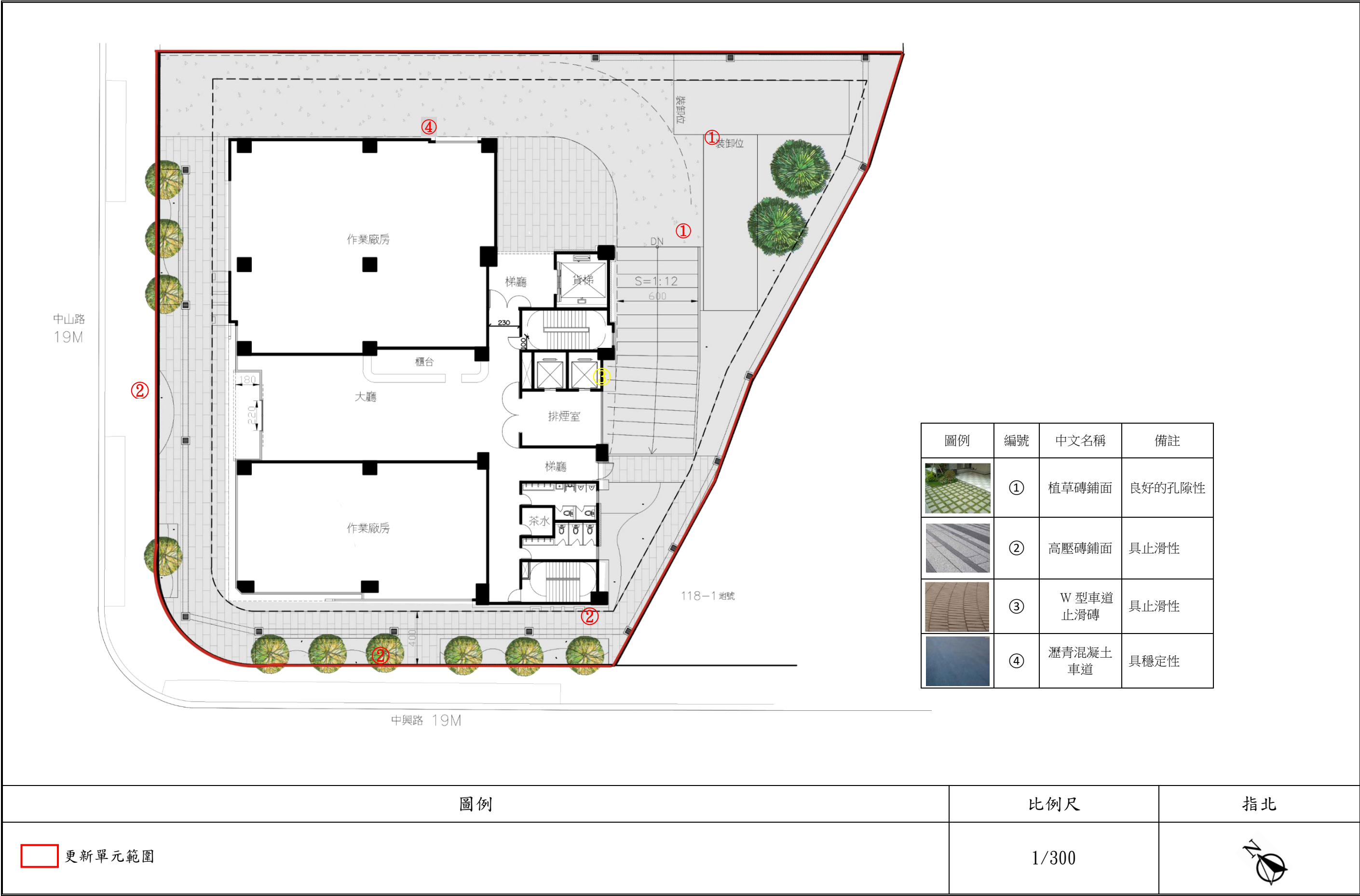
圖12-26 地面層鋪面設計圖
