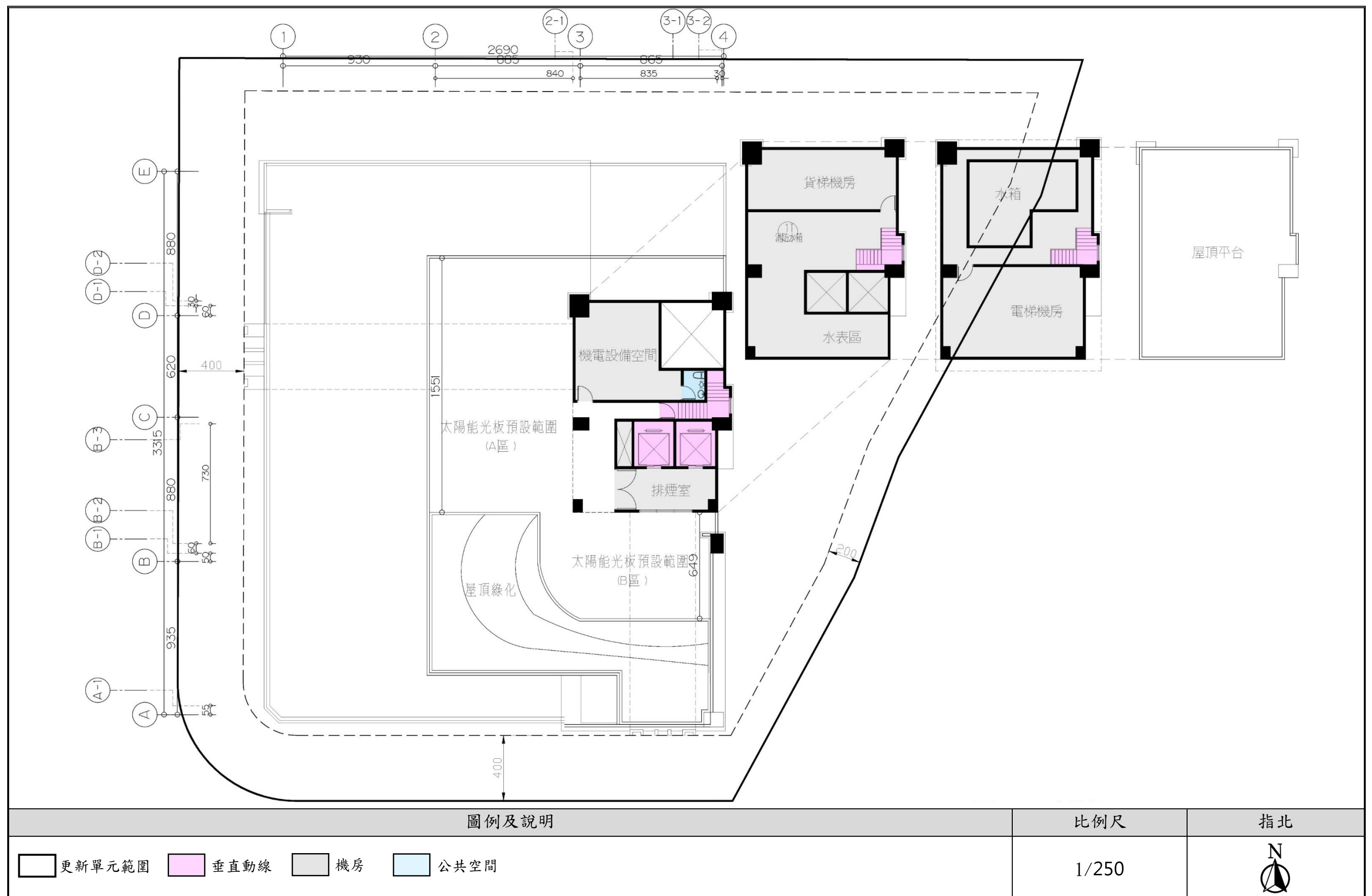
圖11-20 屋頂層及屋凸一至三層平面圖
