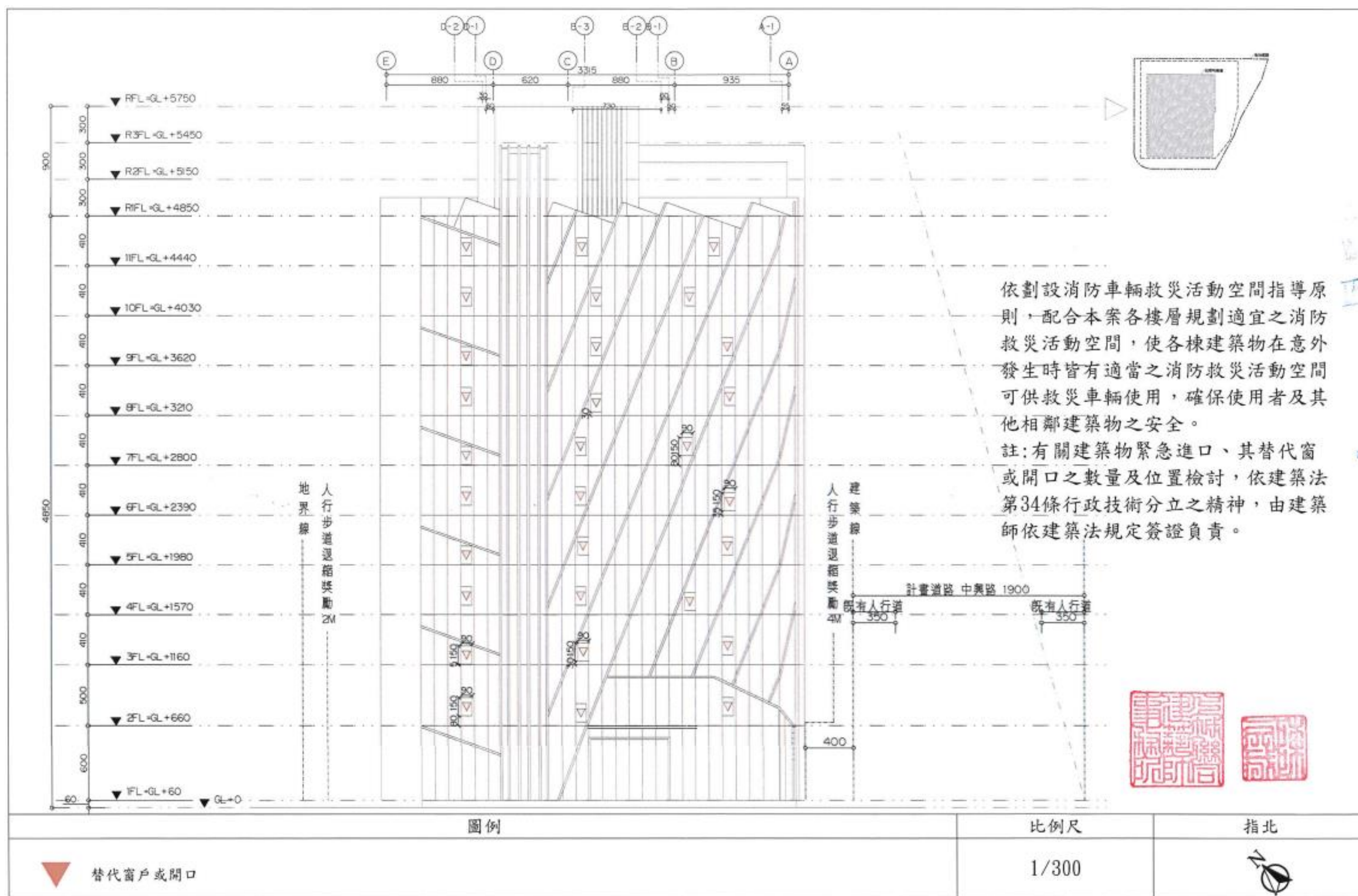
圖6 雲梯車活動空間示意圖(一)
