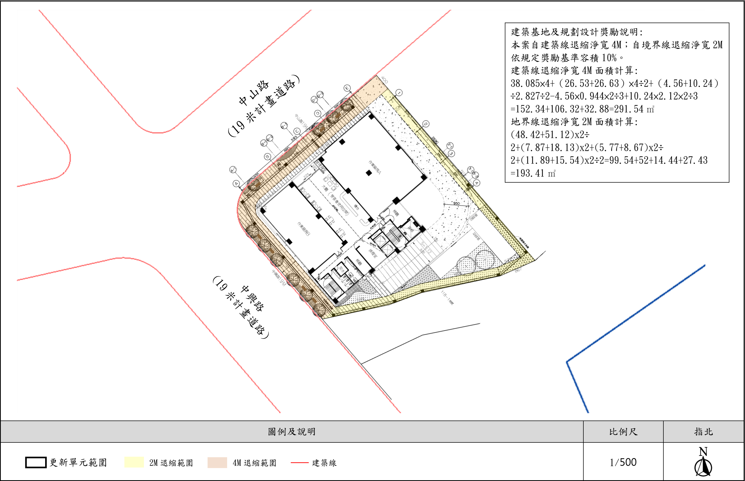
圖10-1 一層規劃設計退縮範圍圖
