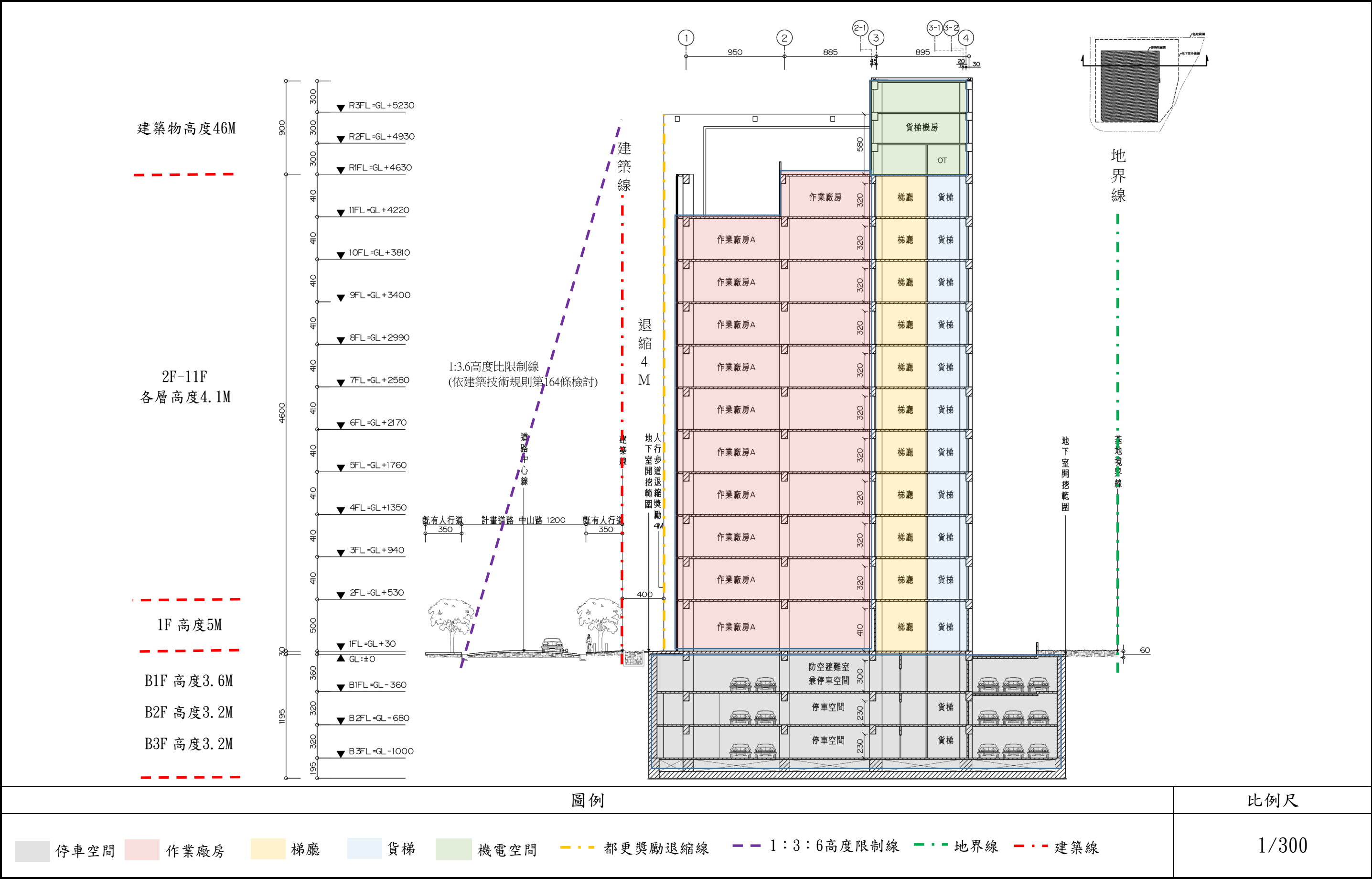
圖12-2 更新後樓層空間用途示意圖
