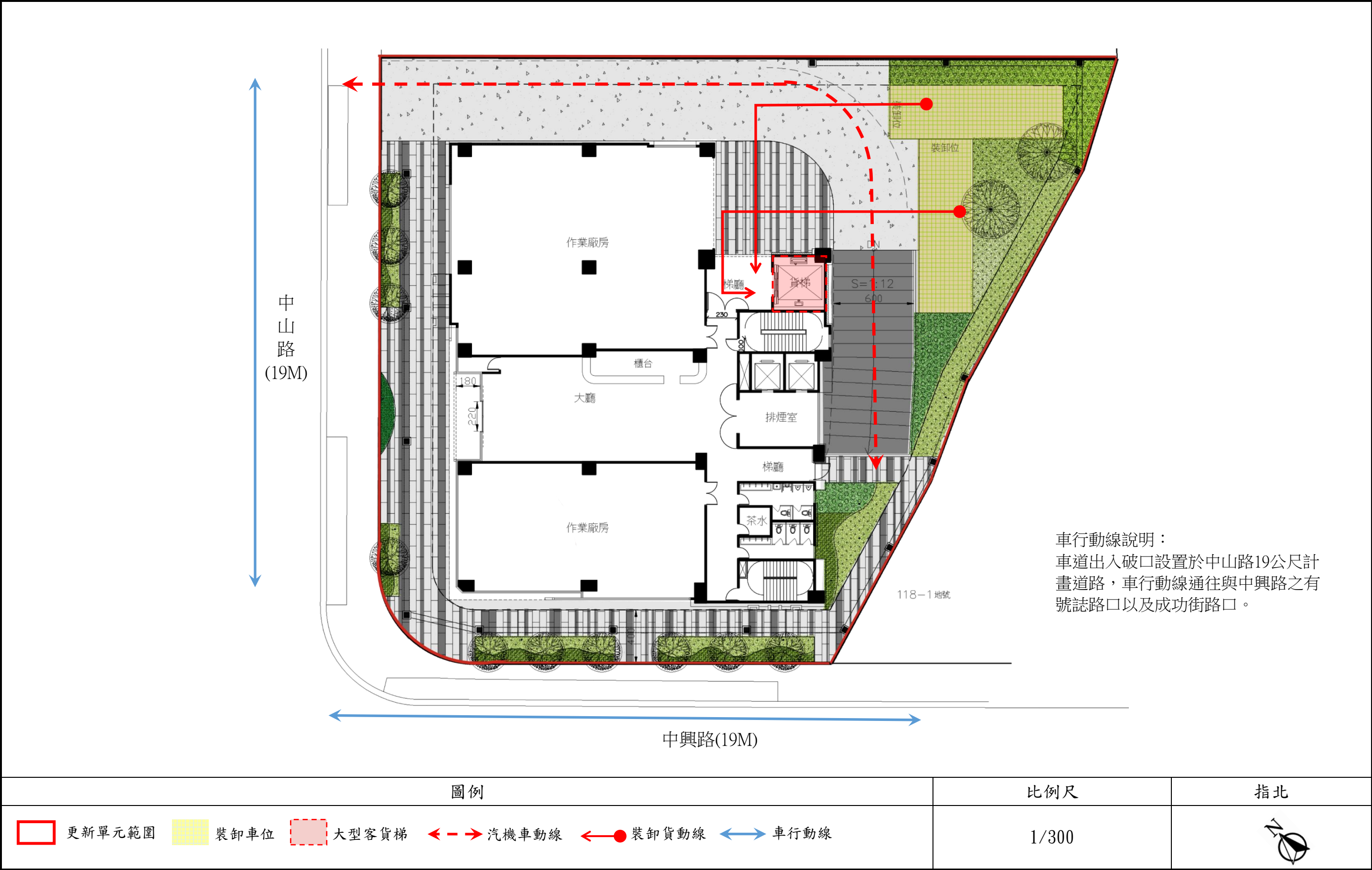
圖12-7 車行動線示意圖
