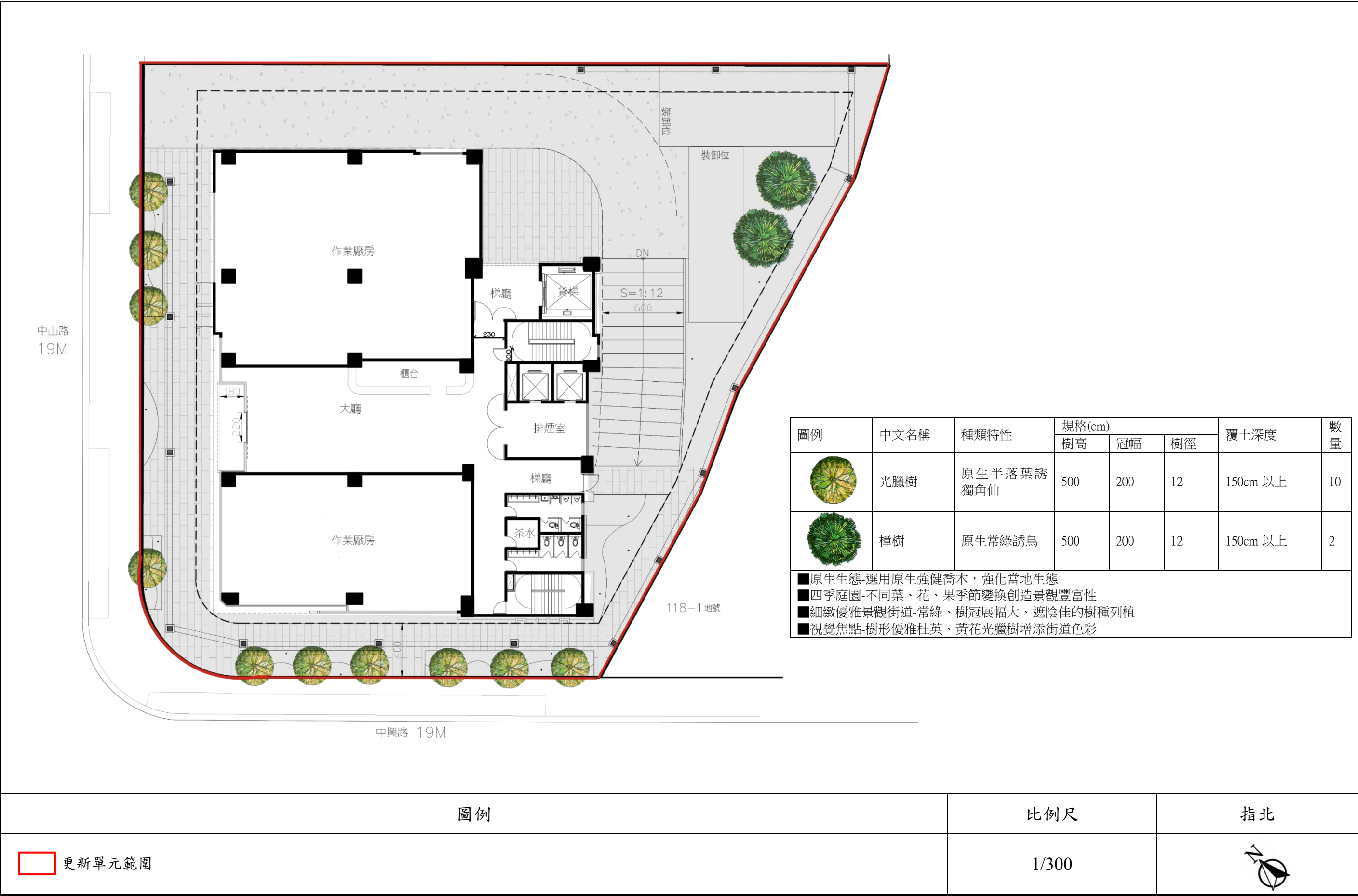
圖12-22 景觀喬木植栽配置圖
