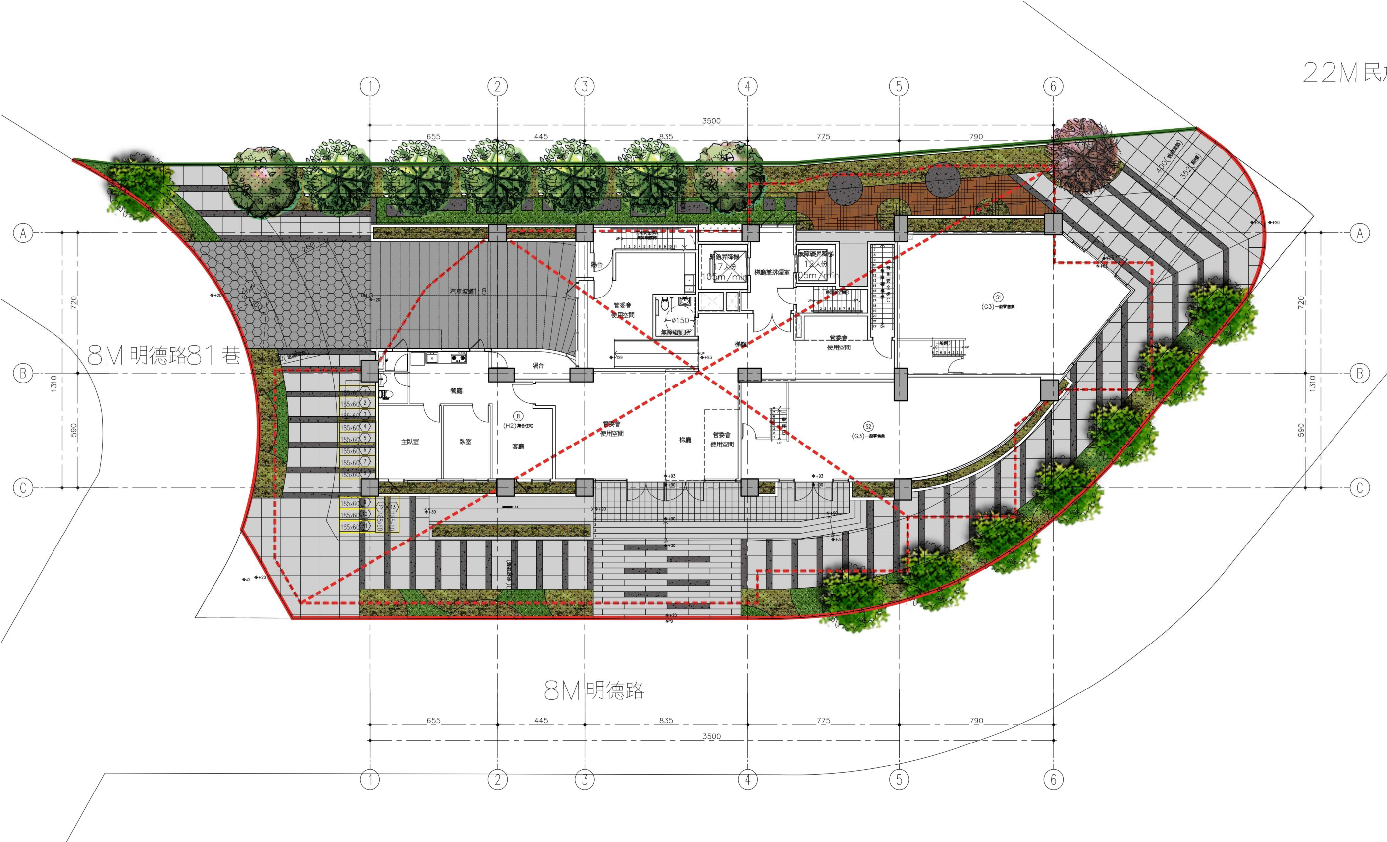
圖 6-7 一層平面圖 (1/200)
