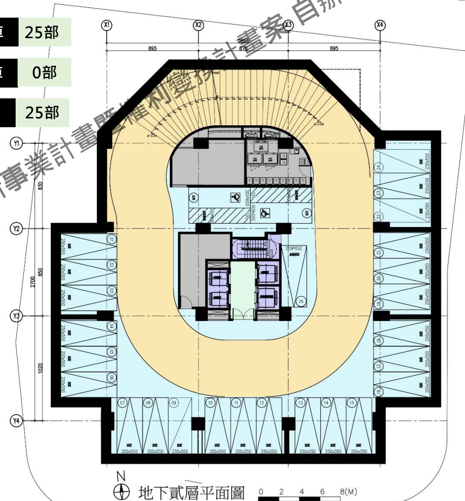
地下二層平面圖
