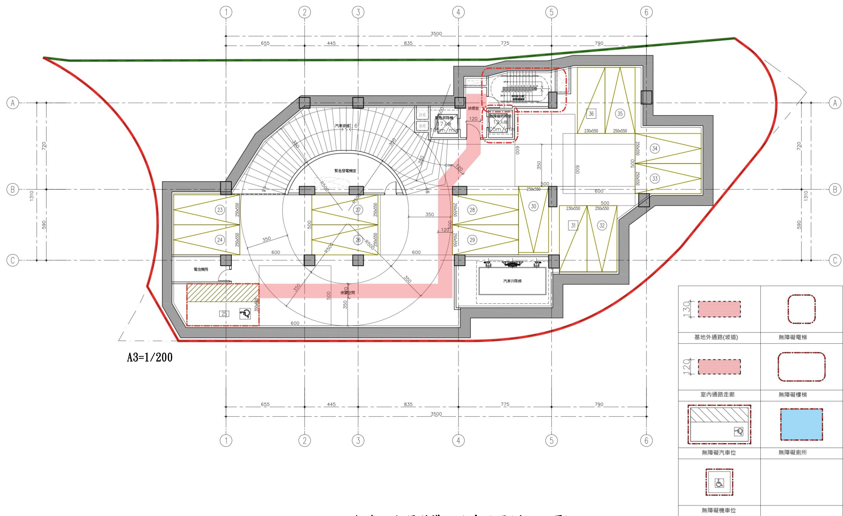
圖 12-13 無障礙空間引導設施系統圖(地下二層)
