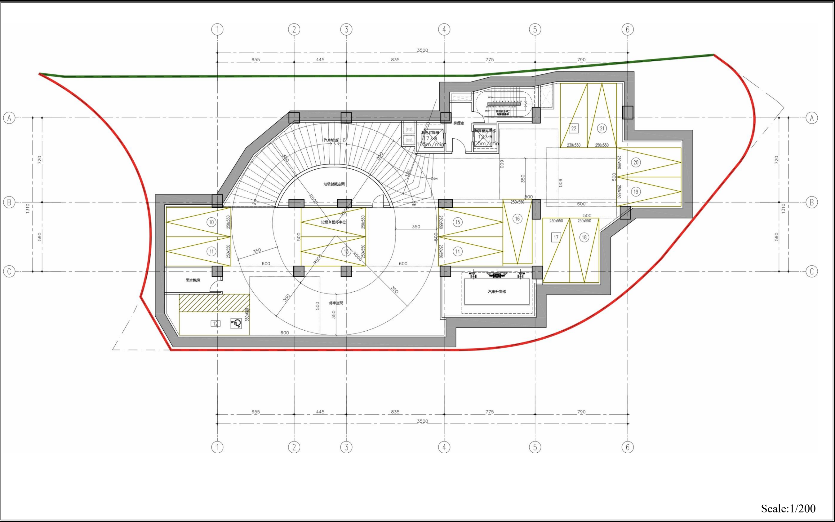
圖 11-17 更新範圍地下三層平面圖
