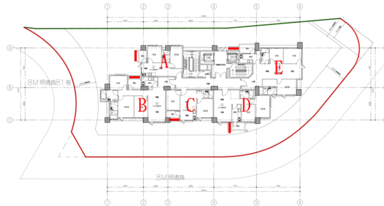
標準層空調配置圖 S:1/400
