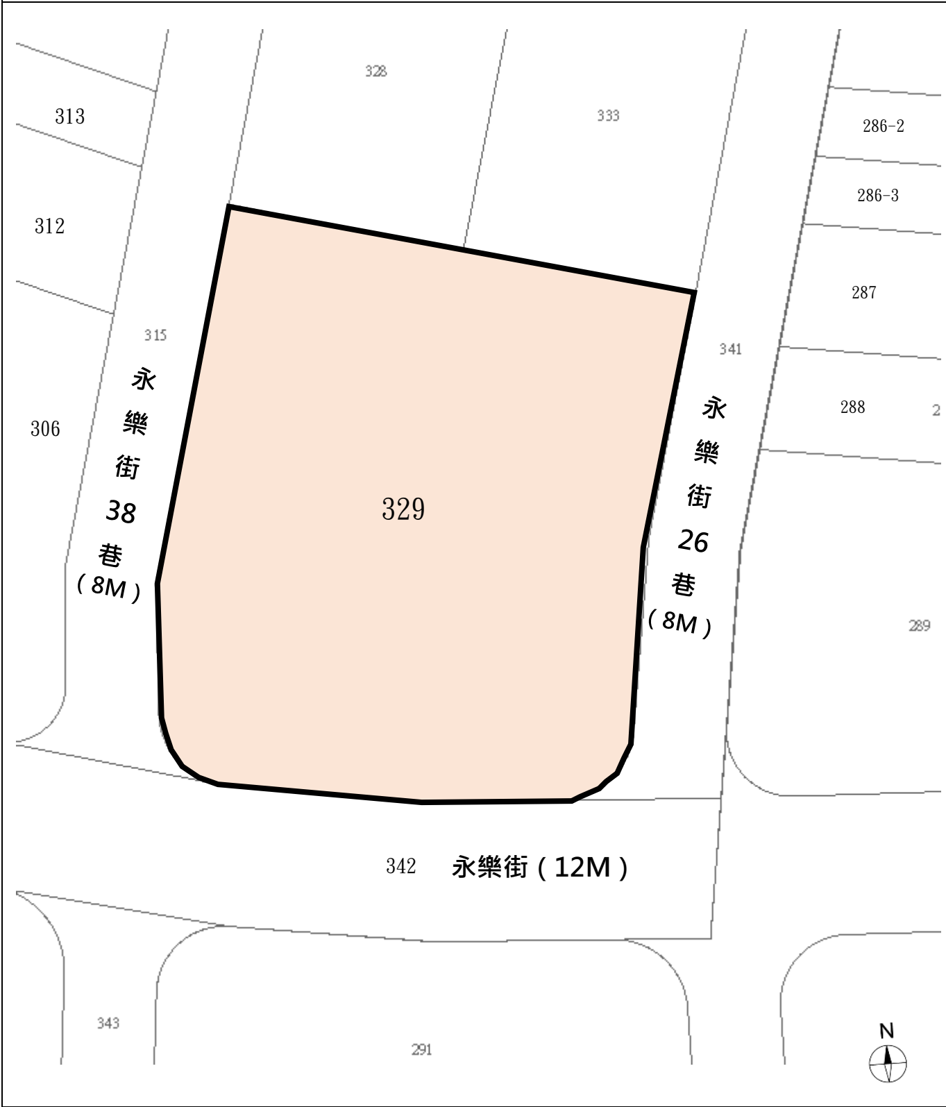
更新單元位置圖 S：1/500
