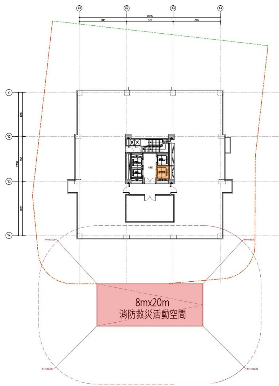
雲梯車救援動線屋突一層平面圖
