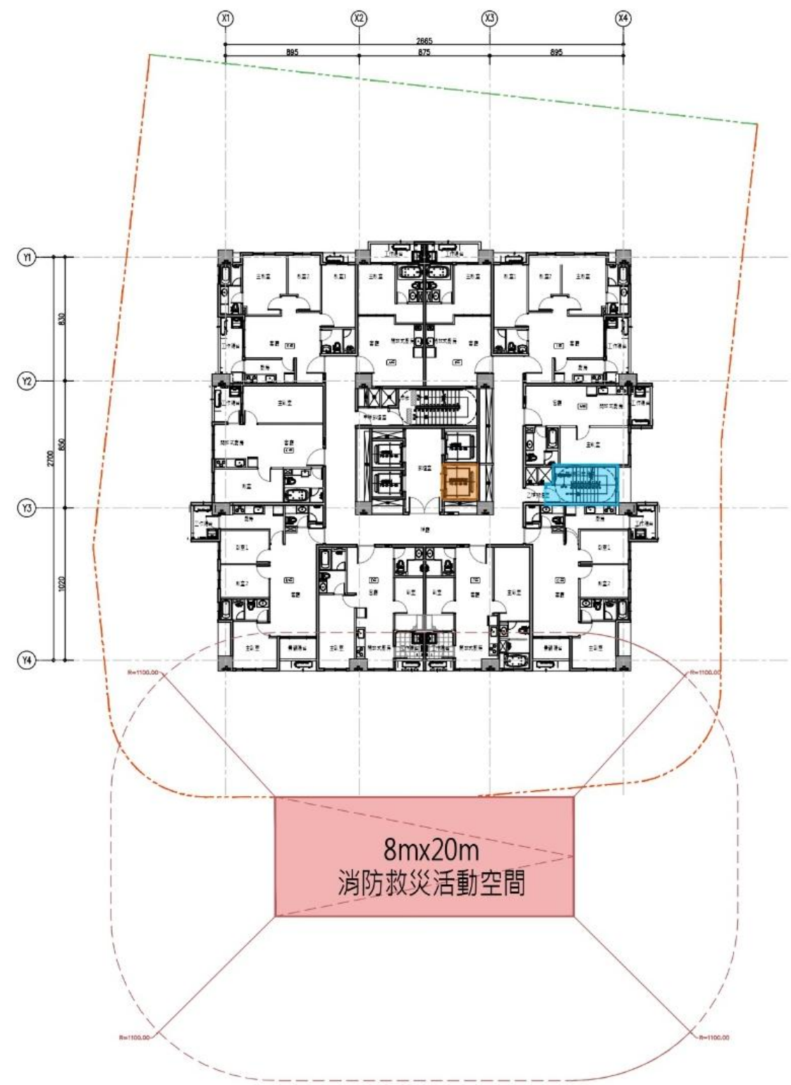
雲梯車救援動線九至十九層平面圖
