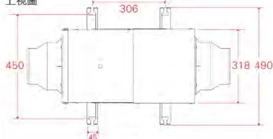
上視圖
