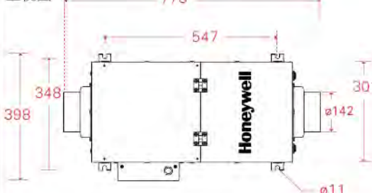
上視圖
