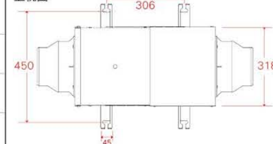
上視圖
