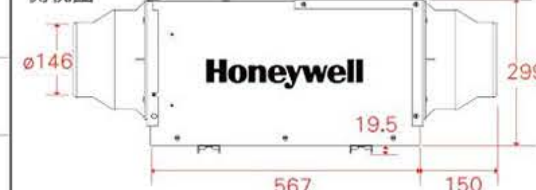
上視圖
