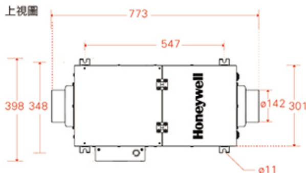
上視圖
