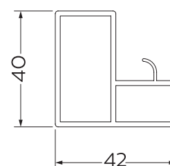
DIMENSIONE PROFILI A PARETE
