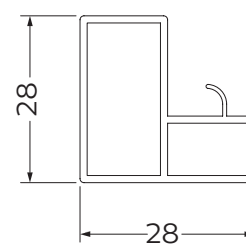
DIMENSIONE PROFILI A PARETE
