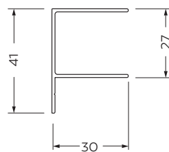
DIMENSIONE PROFILI A PARETE
