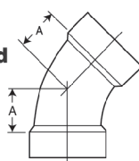
1/8 Bend
