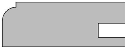
#7015 13/16" x 2 1/4"
