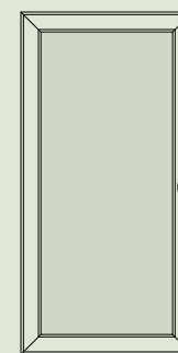
Art. 372042 ANTA lunga per vetro cm. L. 59 SP. 2,8 H. 118
