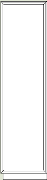
Art. 373074 COL. singola SX. Art. 373075 COL. singola DX. cm. l. 57 p. 37 h. 225
