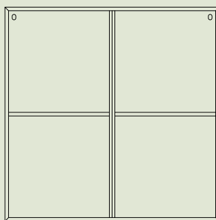
Art. 372049 Struttura PENSILE a cubo 4 vani cm. L. 118 P. 38 H. 118
