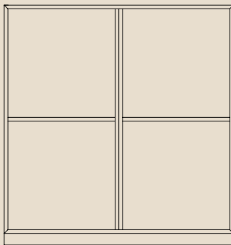
Art. 374120 Colonna 4 vani. cm. L. 118 P. 36 H. 124
