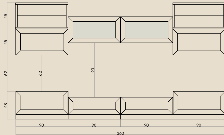
Art. 121062 COMPOSIZIONE cm. L. 360 P. 57/38 H. 200
