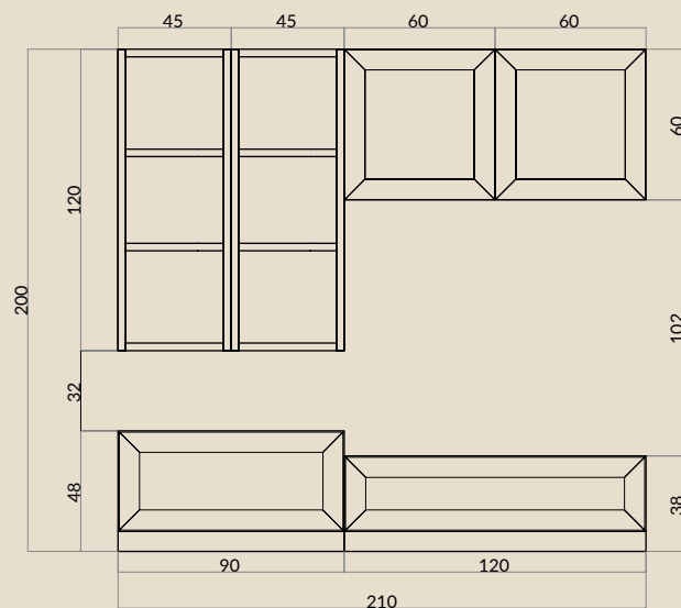
Art. 121056 COMPOSIZIONE. cm. L. 210 P. 57/38 H. 200
