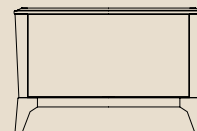
Art. 370535 Base 1 cestone liscio. cm. L. 83,5 P. 56 H. 54,3
