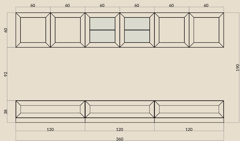
Art. 121066 COMPOSIZIONE cm. L. 360 P. 57/38 H. 190
