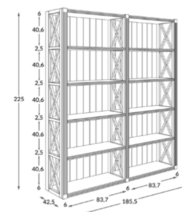
ARTICOLO| H644 Libreria smontabile doppia con fianchi a croce Removable double bookcase with X-shaped sides
