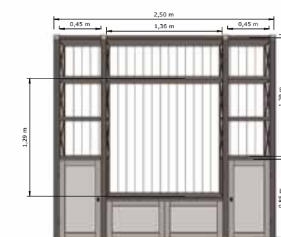
ARTICOLO| H650 Parete con luci led con 2 porte e 2 cassetti. Composition 2 doors and 2 drawers with led. cm. L. 250 H. 225 P. 43 M3 0,6 smontata Kg. 190
