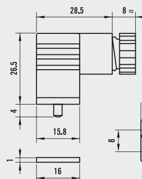
DIN Connector
