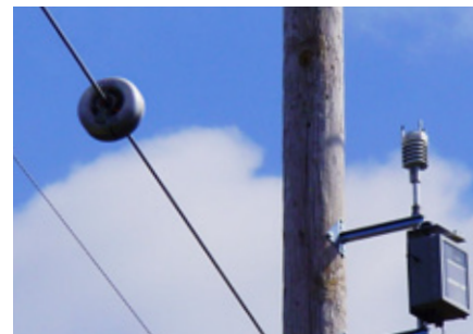
Sistema de medición inalámbrica PowerDonut, de variables en líneas de transmisión eléctrica AT/MT y estación meteorológica con DLR.
