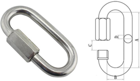
QUICK LINK 快速连接环
