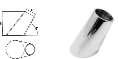
AISI316 STAINLESS STEEL 60°STANCHION BASE 316不锈钢斜60° 旗杆座
