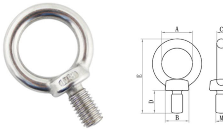
JIS1168 EYE SCREW JIS1168 日式吊环螺丝
