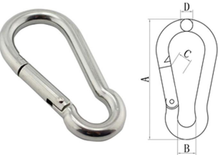
CARABINER HOOK 登山扣
