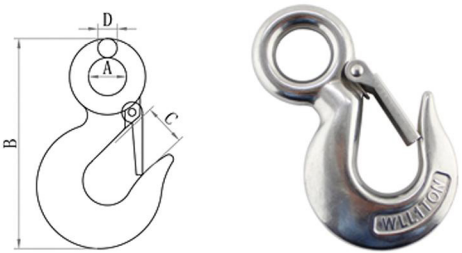
S320 CRANE HOOK S320 货钩
