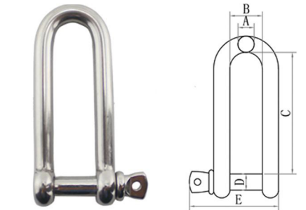
LONG D SHACKLE 长D卸扣
