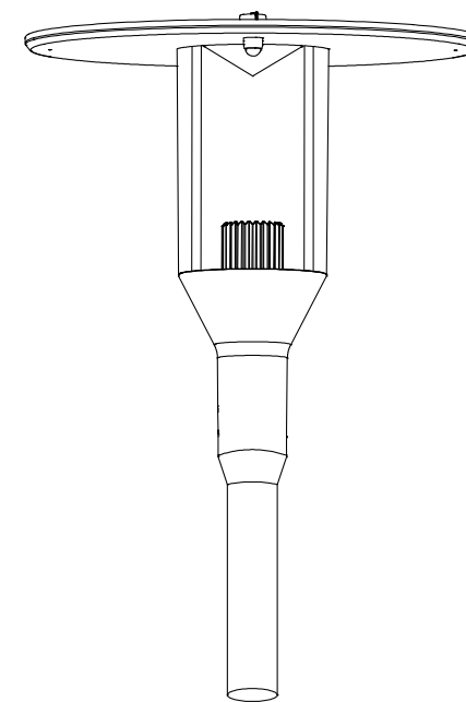
Ø60mm pole
