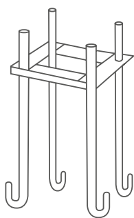
Nedstøbningsbeslag
