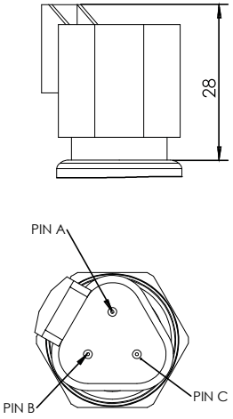
DEUTSCH DT04-3P IP67
