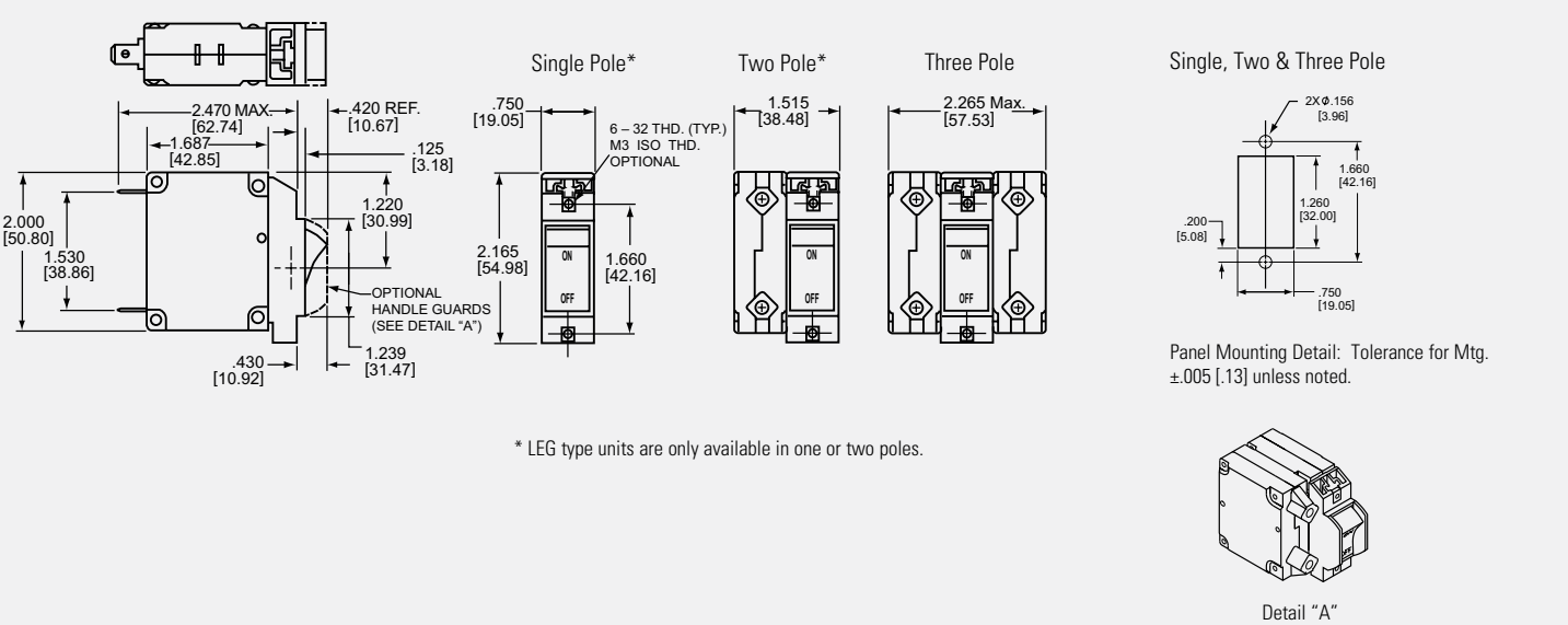
IAGZX/IUGZX/IEGZX/CEGZX/LEGZX
