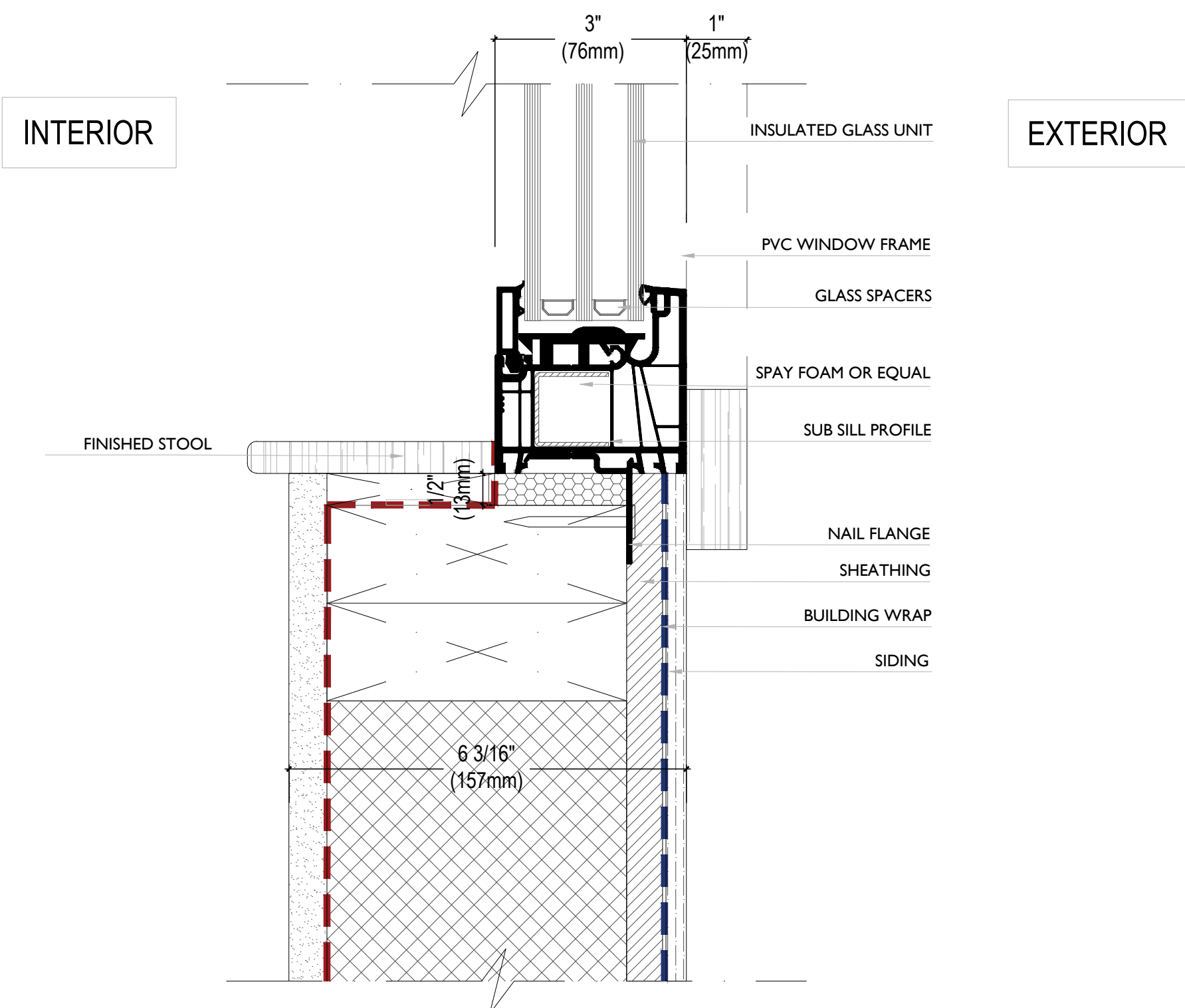
03 WINDOW SILL DETAIL A-02 SCALE: 6"=1'-0"
