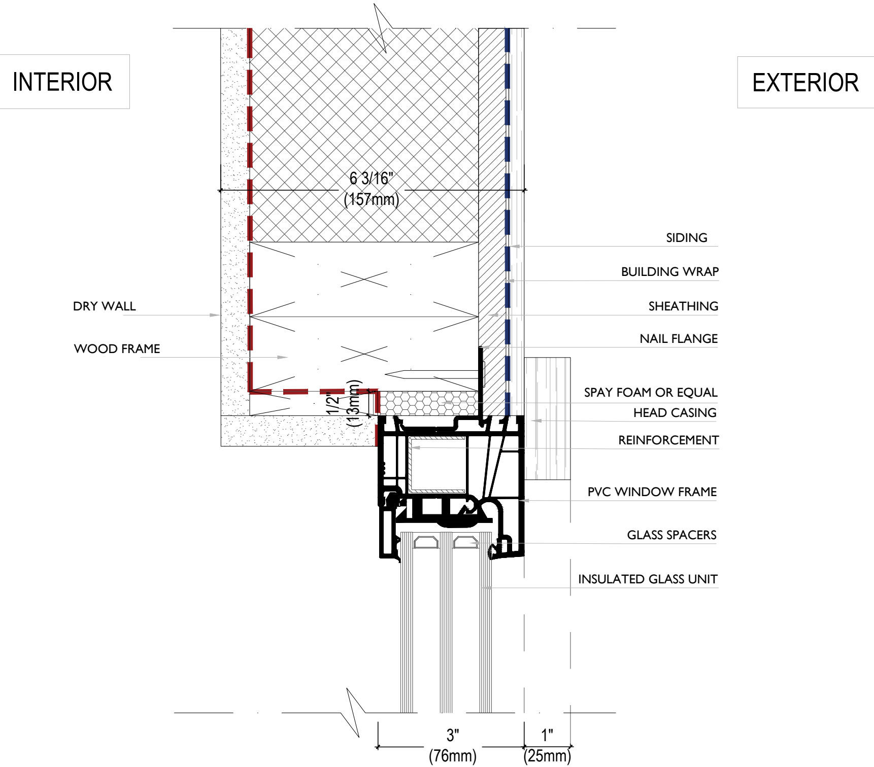
01 WINDOW HEAD DETAIL A-02 SCALE: 6"=1'-0"
