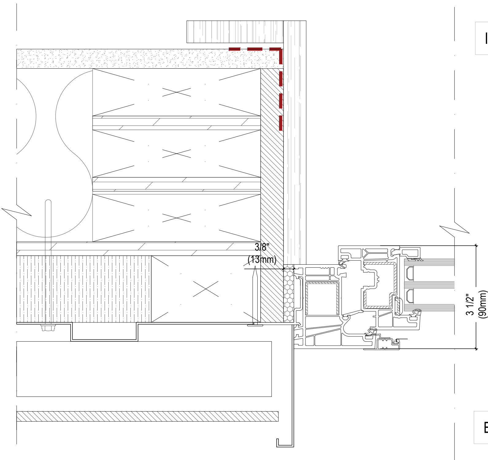
02 WINDOW JAMB DETAIL A-03 SCALE: 6"=1'-0"
