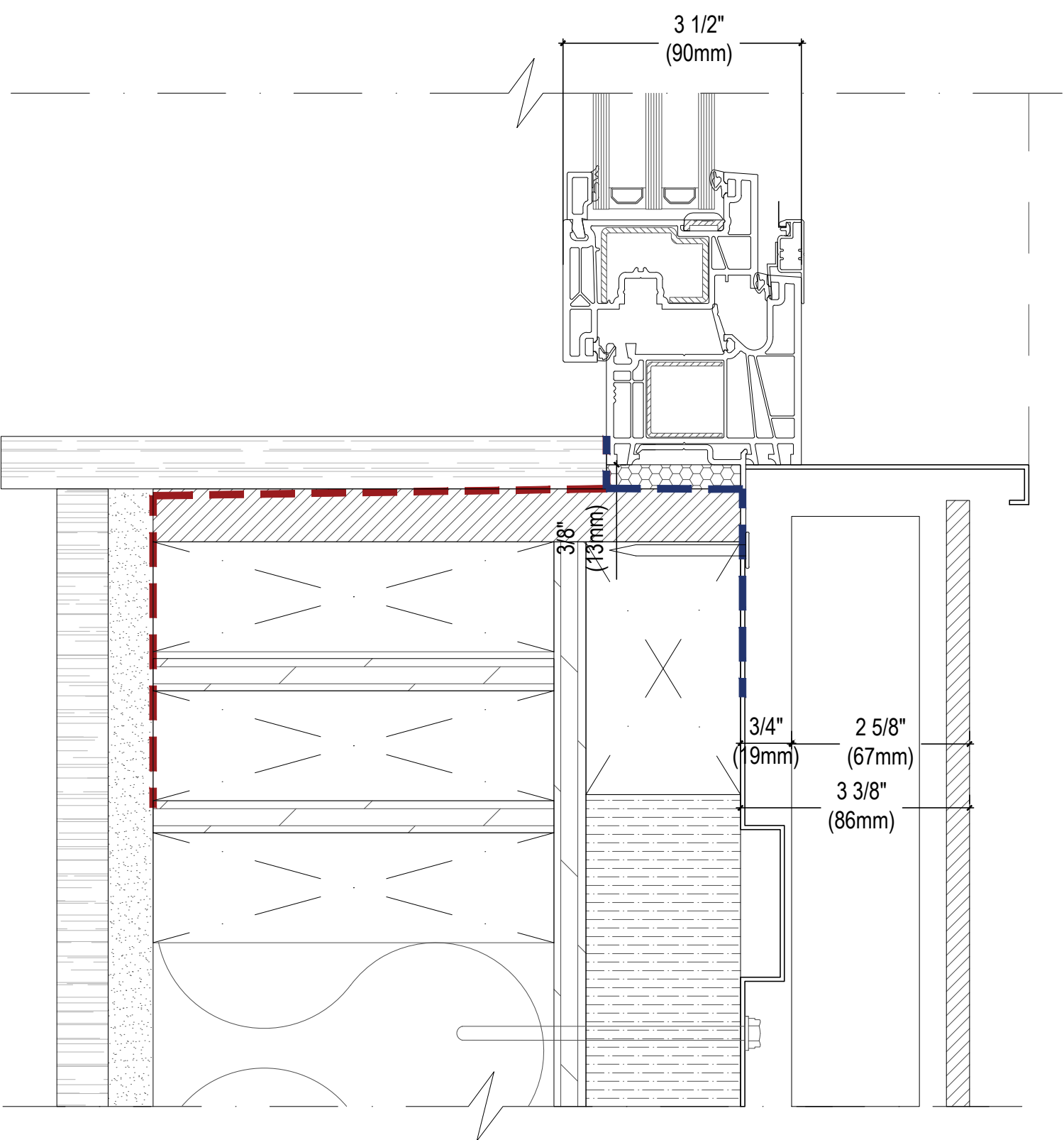
03 WINDOW SILL DETAIL A-03 SCALE: 6"=1'-0"
