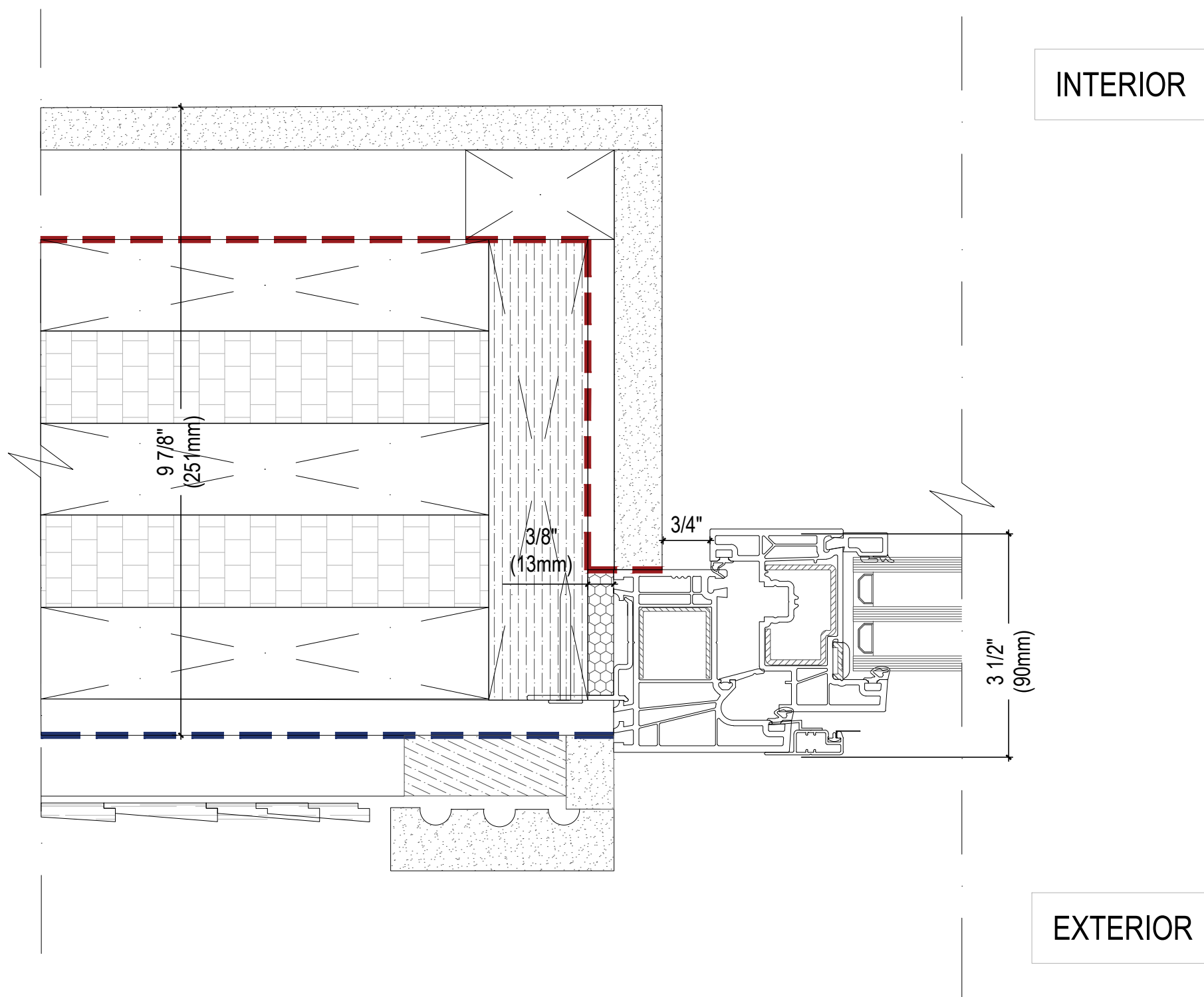
02 WINDOW JAMB DETAIL A-04 SCALE: 6"=1'-0"
