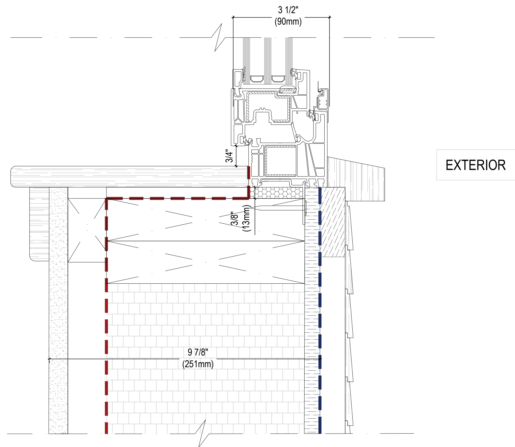
03 WINDOW SILL DETAIL A-04 SCALE: 6"=1'-0"
