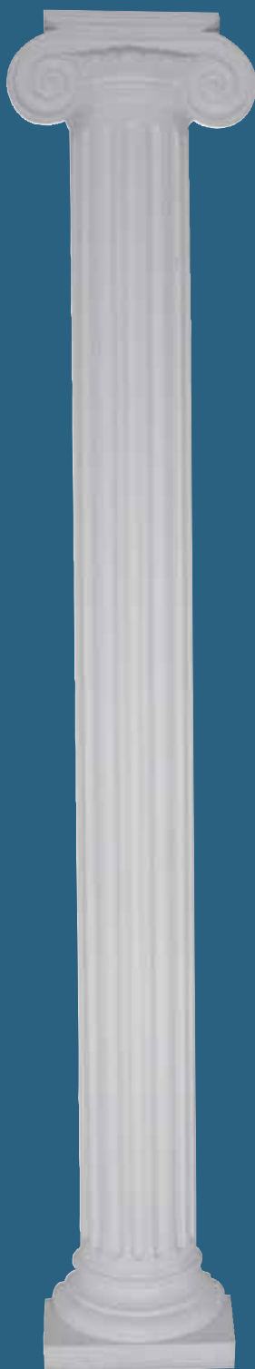
Art. 1800 CAPITELLO 41x28cm H. 18cm FUSTO H. variabile Ø 20cm Base largh. 33x33cm H. 18cm
