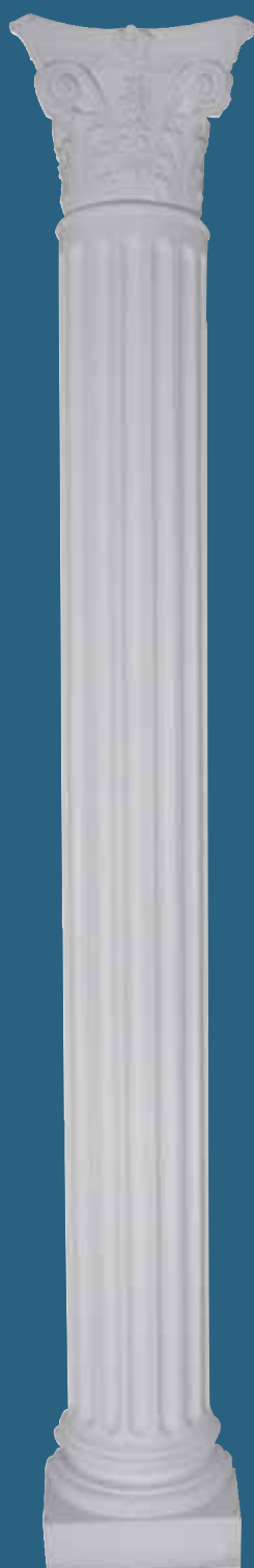
Art. 1833 CAPITELLO 37x37cm H. 29cm FUSTO H. variabile Ø 22cm Base largh. 30x30cm H. 21cm
