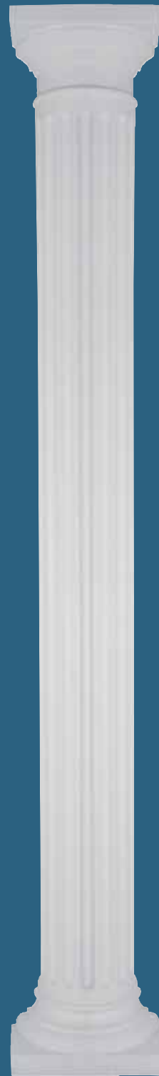
Art. 1801 CAPITELLO 31,5x31,5cm H. 19,5cm FUSTO H. variabile Ø 20cm Base largh. 33x33cm H. 18cm
