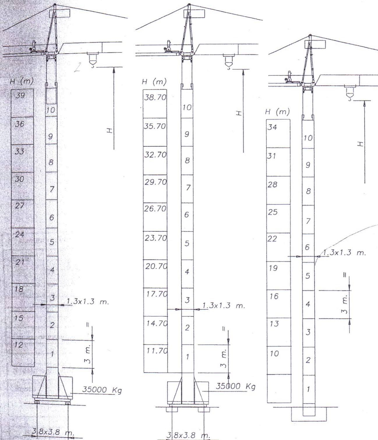
Versione gru traslante
