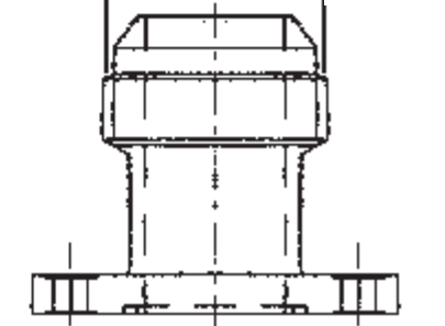
JIC 16 (-16AN)
