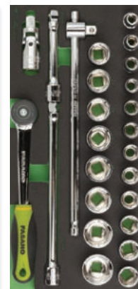
FG 100/45D: Modulo 6 giraviti taglio e croce FG 100/21B: Modulo chiavi a bussola esagonali da 1/2" FG 100/21TX: Modulo utensili con impronta Torx da 1/4" e 1/2"
