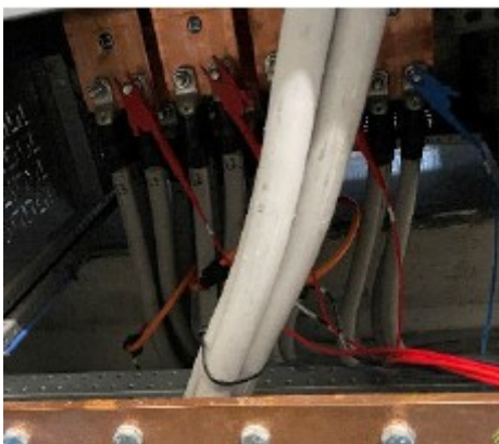
Installazione di misura. L'immagine mostra un dettaglio del collegamento dello strumento al punto di misura.
