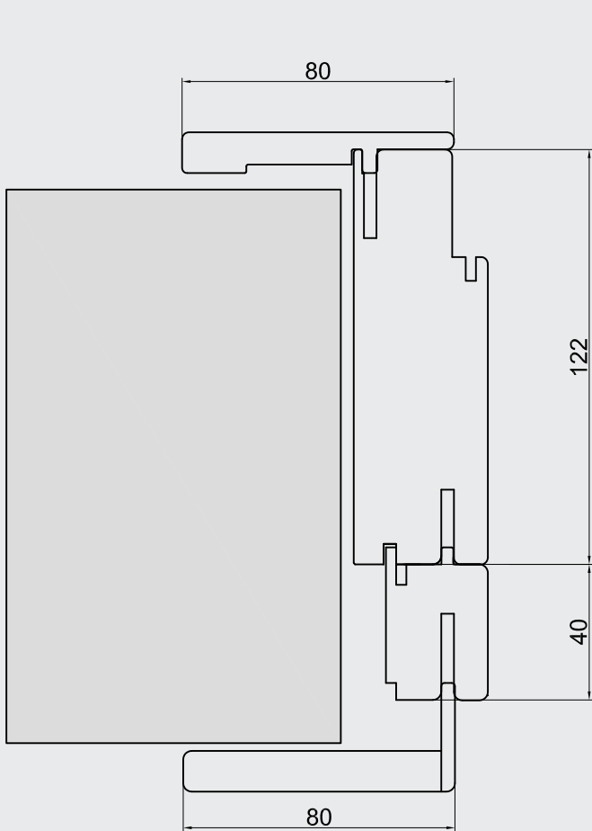
Allargamento per muro spesso da 15.5 a 17 cm
