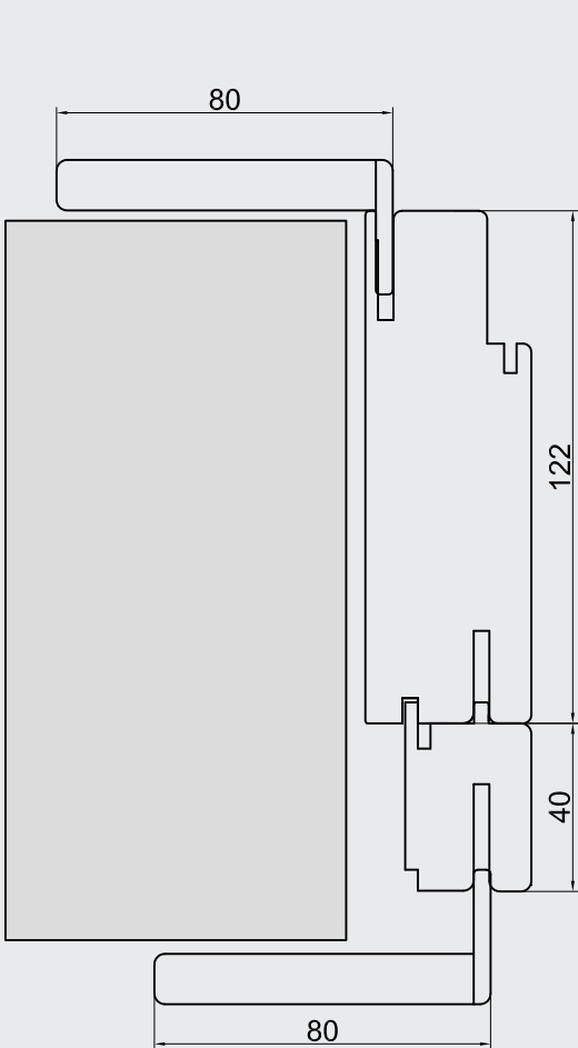
Allargamento per muro spesso da 16 a 17.5 cm
