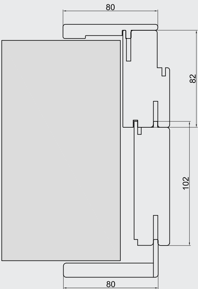
Allargamento per muro spesso da 17.5 a 19 cm
