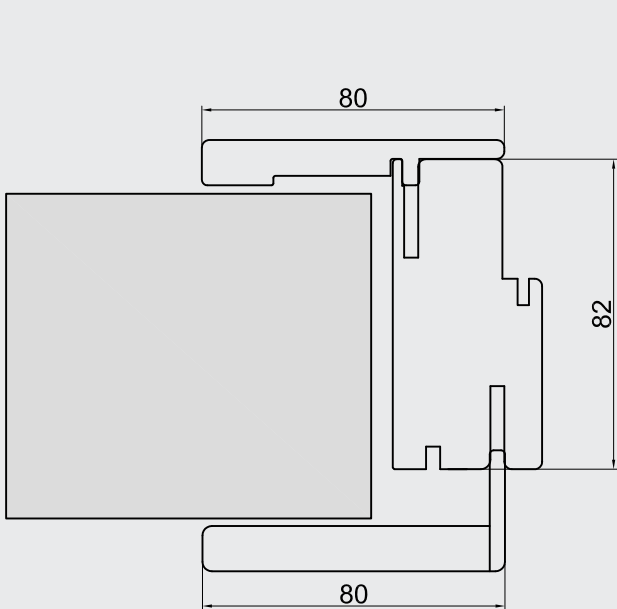
Per muro spesso da 7.5 a 9 cm For thickness from 7.5 to 9 cm Elargissement pour épaisseur de mur de 7.5 à 9 cm Expansión pared de 7.5 a 9 cm
