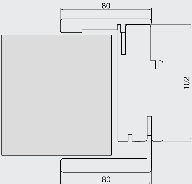
Per muro spesso da 9.5 a 11 cm For thickness from 9.5 to 11 cm Elargissement pour épaisseur de mur de 9.5 à 11 cm Expansión pared de 9.5 a 11 cm
