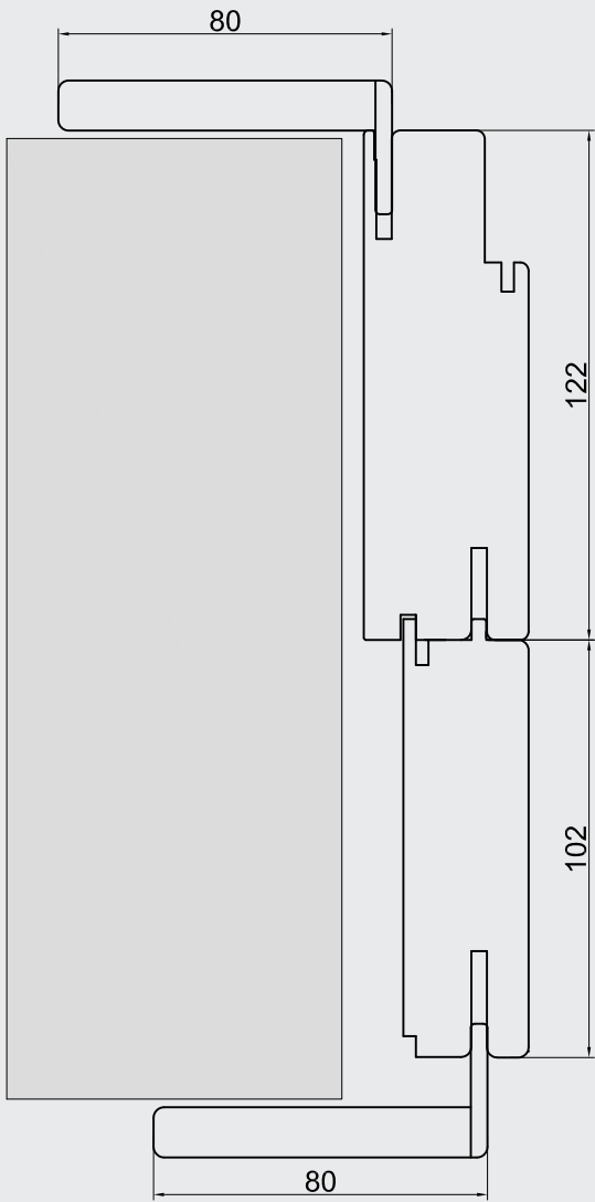
Allargamento per muro spesso da 22 a 23.5 cm
