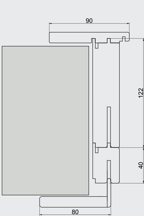
Allargamento per muro spesso da 15.5 a 17 cm
