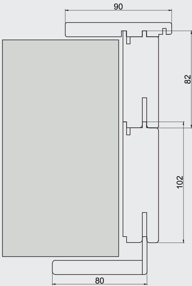
Allargamento per muro spesso da 17.5 a 19 cm
