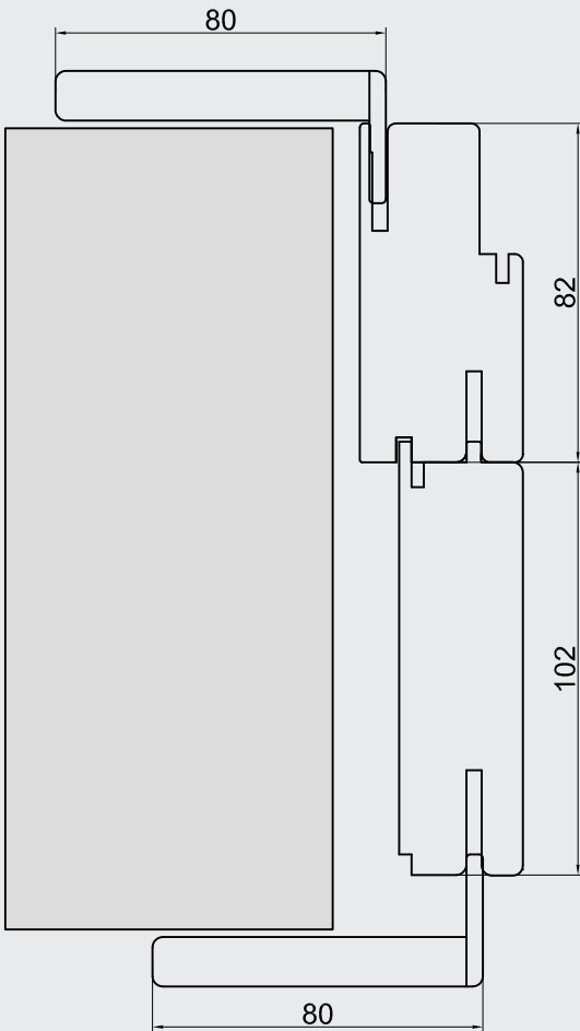
Allargamento per muro spesso da 18 a 19.5 cm
