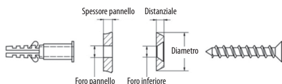
DISTANZIALE
