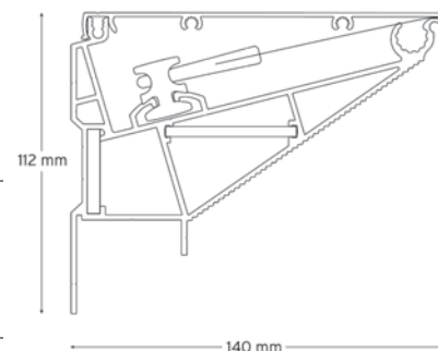
SEZIONE PROFILO PRINCIPALE
