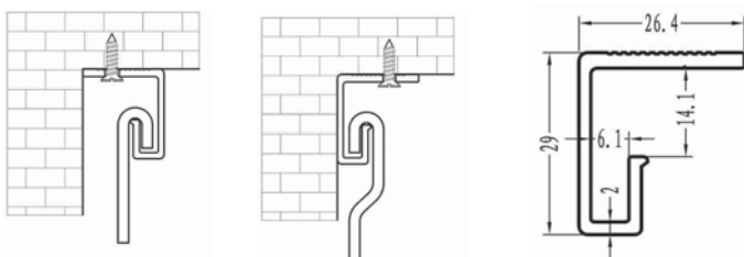
Montaggio nascosto
