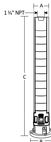
Acoplamiento NEMA 6"
