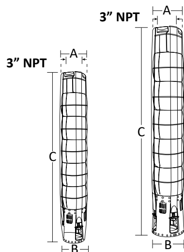
Acoplamiento NEMA 4"
