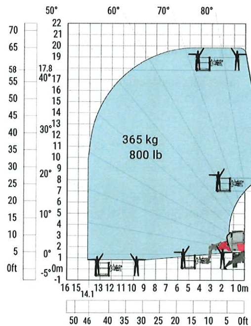
Rotazione su stabilizzatori con cestello da 365 kg
