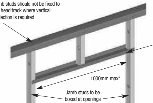
Fig. 1 Door Opening
