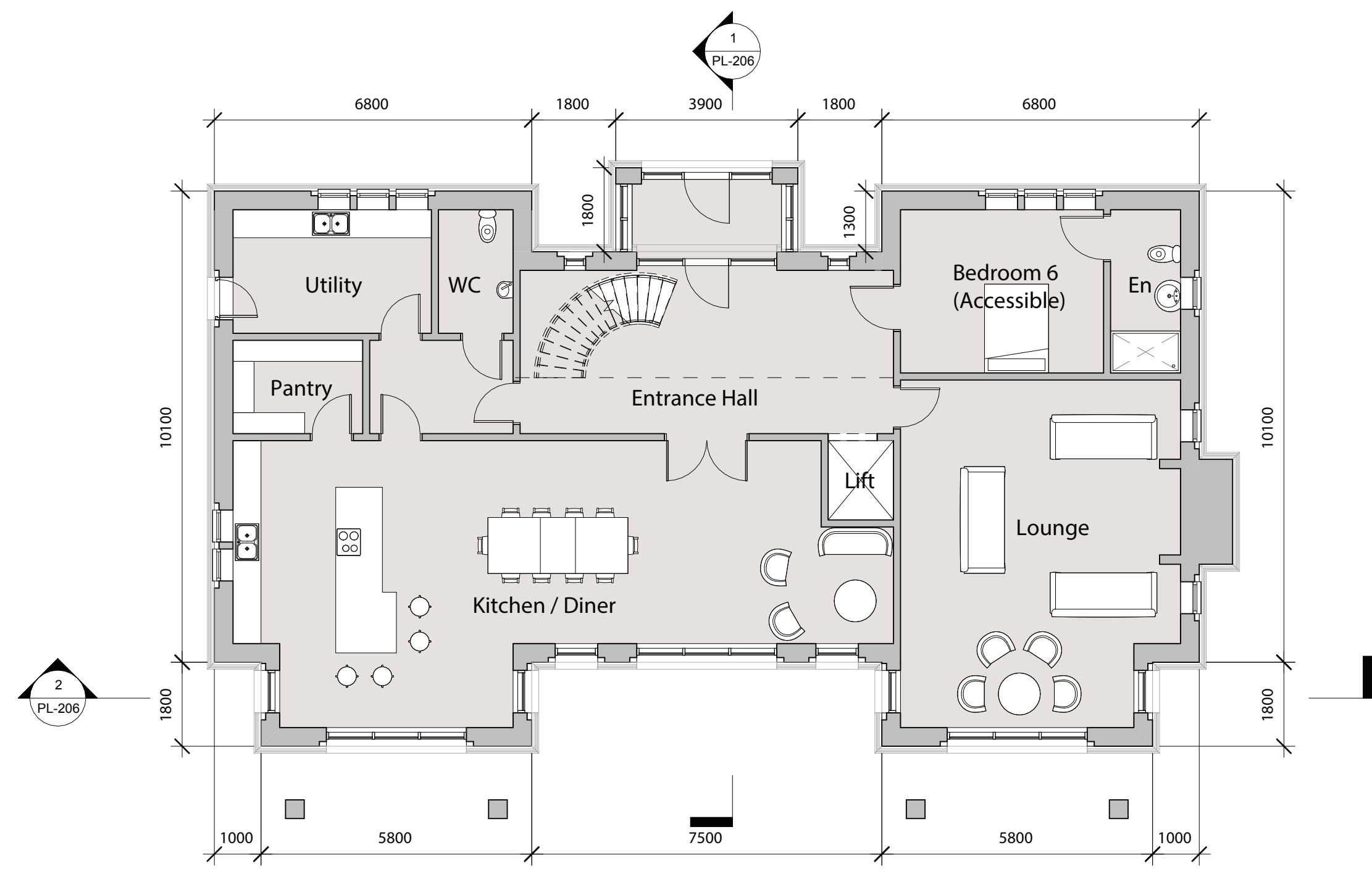
0_Ground Floor 1 : 100
