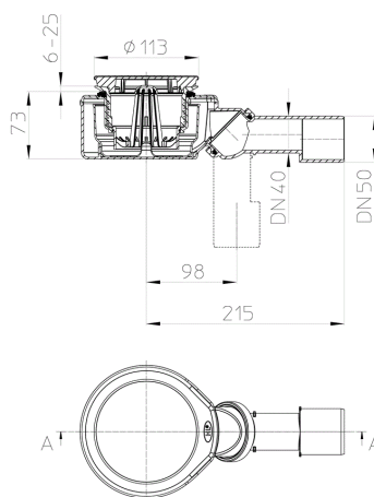
Schnitt A-A
