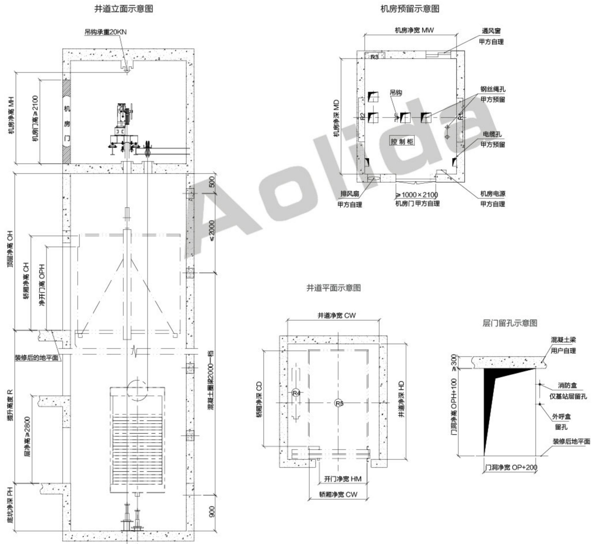
AEP200 Small machine room bed elevator parameter table
