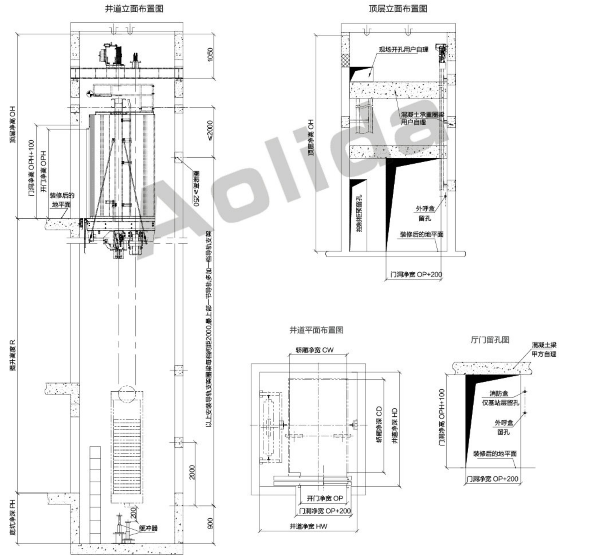
AEP320 Machine roomless bed elevator parameter table
