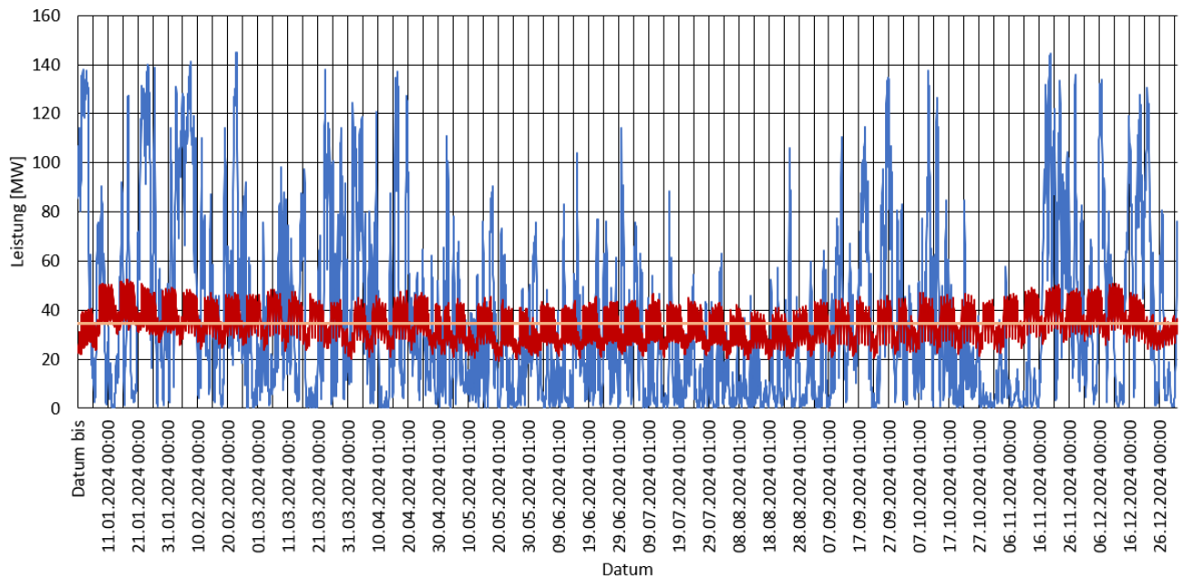
27 Windräder N175-6.8 AÖ-Forst Windstromerzeugung 2024 und Verbrauchskurve 2024 Datenquelle Windmessung Qair, TransnetBW. Berechnung und Darstellung: W. Fritz
