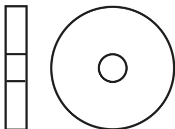
Scheiben für Holzverbindungen, mit Rundloch DIN 440-R blank, galvanisch verzinkt
