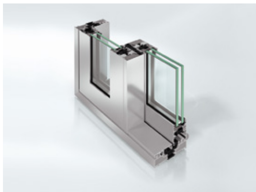
Schüco ASE 60
