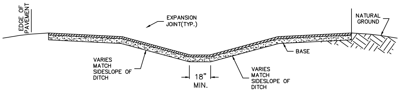
SECTION A-A
