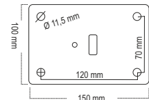
Abmessung der Fußplatte 8 mm dick
