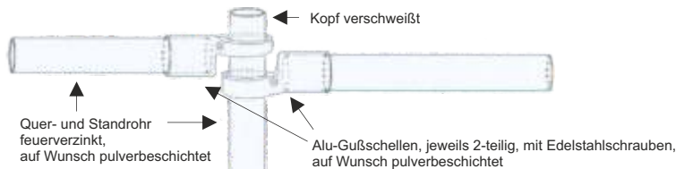
Montagebeispiel starres Geländer
