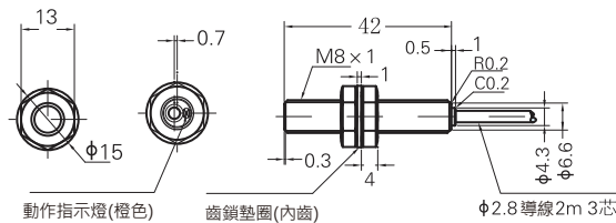
動作指示燈(橙色) 齒鎖墊圈(內齒) φ2.8導線2m 3芯
