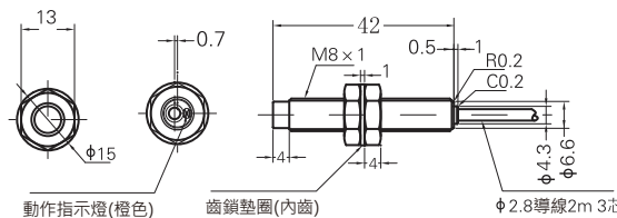
動作指示燈(橙色) 齒鎖墊圈(內齒) φ2.8導線2m 3芯
