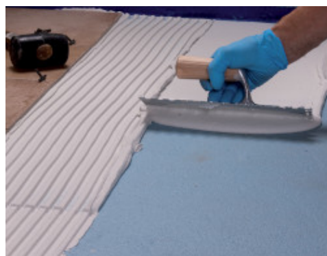
Incollaggio delle piastrelle su Mapelastich AquaDefense Zero
