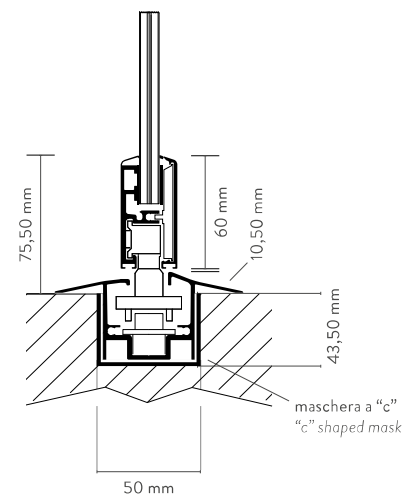
sezione con guida inferiore incassata e maschera a "c" section with lower embedded profile and "c" shaped mask
