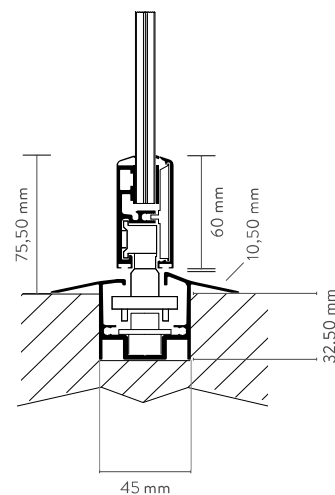
sezione con guida inferiore incassata section with lower embedded profile
