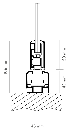
sezione con guida inferiore esterna section with lower external profile
