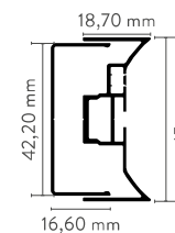
profilo laterale con compensazione a parete side wall profile with compensation
